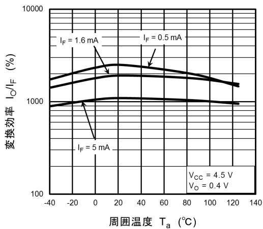
图 12.2.9 I_O/I_F - T_a
