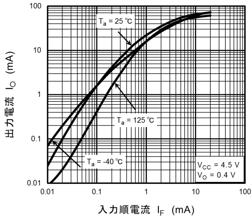
图 12.2.7 I_O - I_F
