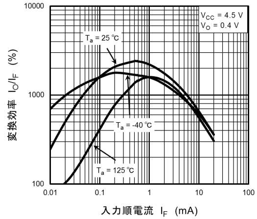
图 12.2.8 I_O/I_F - I_F
