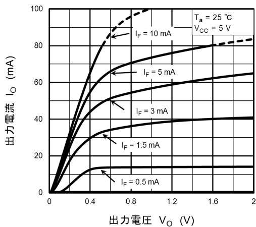
图 12.2.11 I_O - V_O
