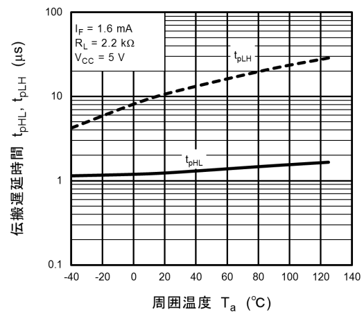
图 12.2.12 t_{pHL}, t_{pLH} - T_a
