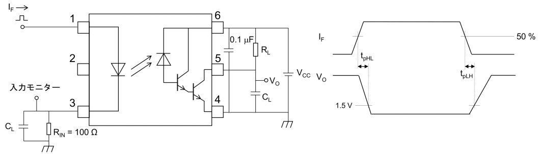
図 12.1.1 伝搬遅延時間測定回路, 波形
