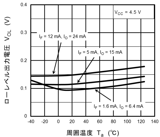
図 12.2.6 V_{OL} - T_a
