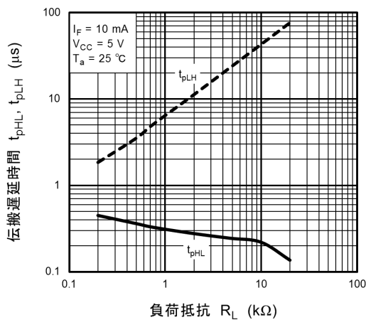
図 12.2.17 t_{pHL}, t_{pLH} - R_L
