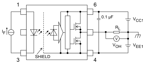
図 13.1.3 V OH 測定回路
