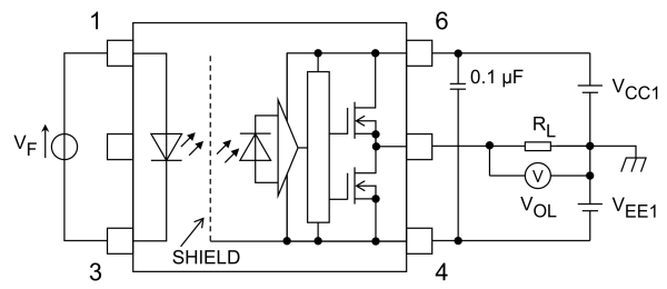
図 13.1.4 V OL 測定回路
