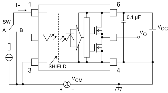
図 13.1.8 コモンモード過渡耐性測定回路, 波形
