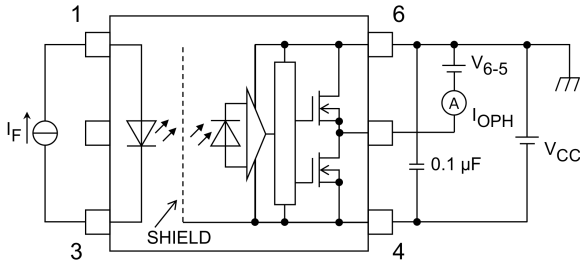
図 13.1.1 I OPH 測定回路
