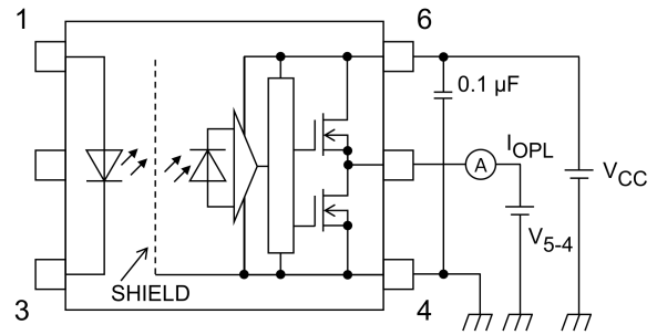
図 13.1.2 I OPL 測定回路
