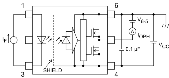
図 13.1.1 I OPH 測定回路
