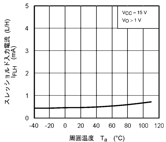
図 13.2.4 I_{FLH} - T_a
