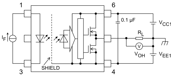
図 13.1.3 V OH 測定回路
