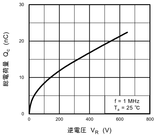
図 9.5 Q_c - V_R
