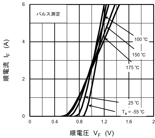
図 9.1 I_F - V_F
