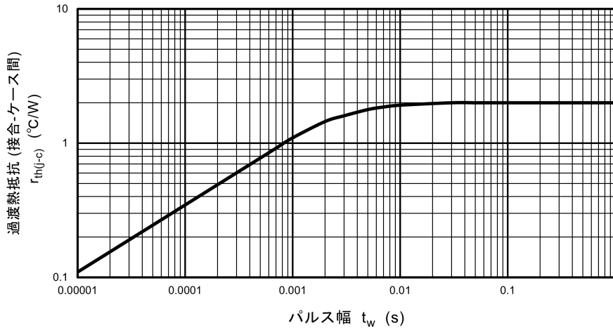
図 9.6 r_{th(j-c)} - t_w (最大値 (保証値))
