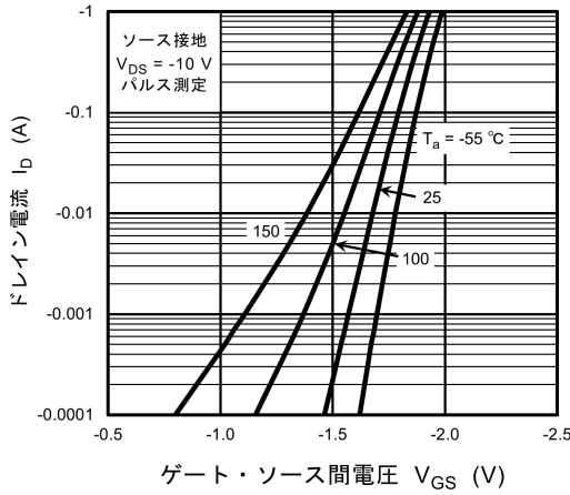
図 8.7 I_D - V_{GS}
