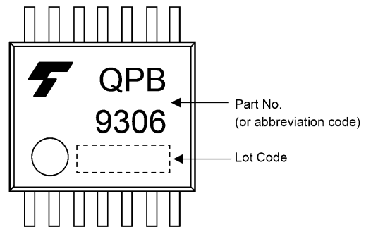
図 6.2 TSSOP14
