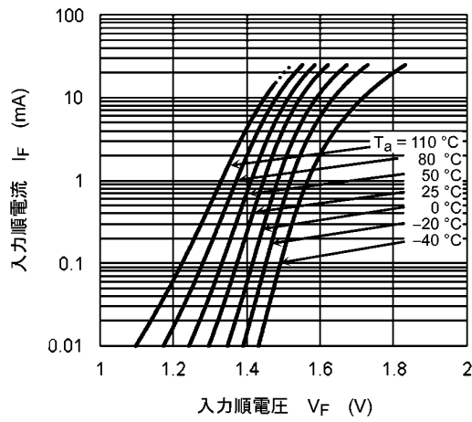
図 13.2.1 I_F - V_F
