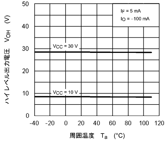
図 13.2.8 V_{OH} - T_a
