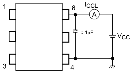
图 13.1.6 I CCL 测定回路
