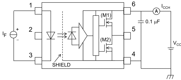
図 13.1.5 I CCH 測定回路
