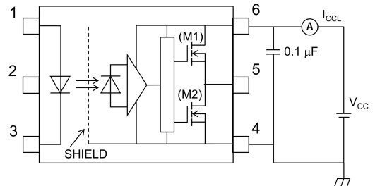
図 13.1.6 I CCL 測定回路
