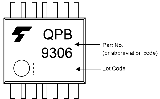
Fig. 6.2 TSSOP14
