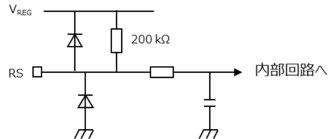
图 6.3 等価回路 (3)
