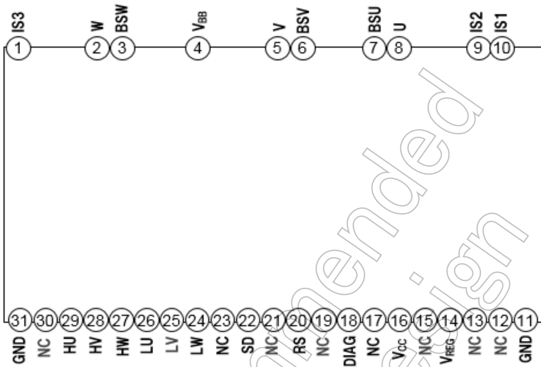
図 5.1 端子配置図
