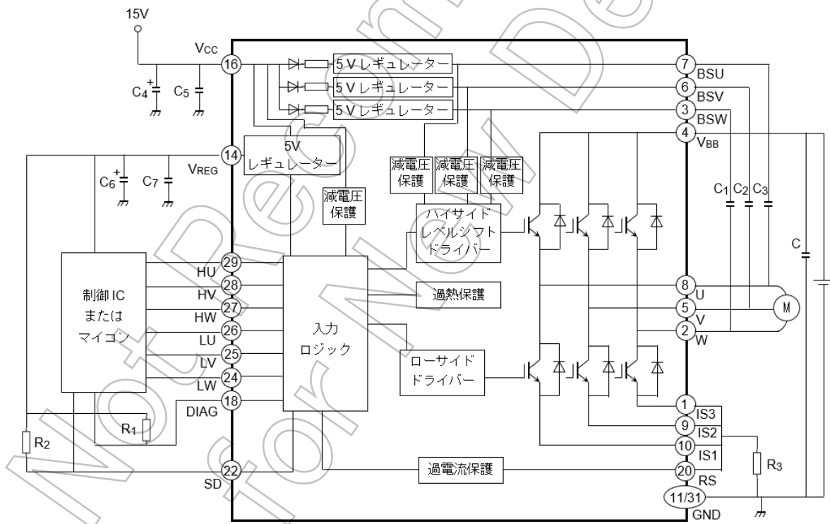
図 12.1 応用回路例
