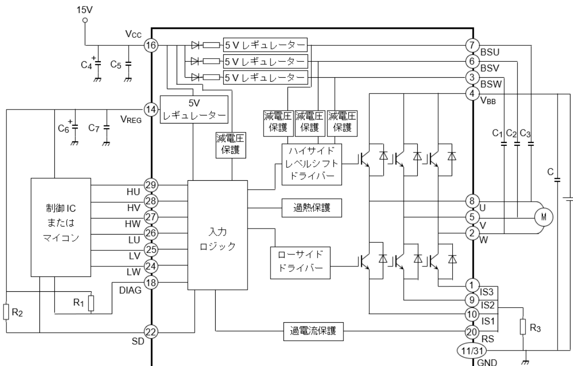
図 12.1 応用回路例
