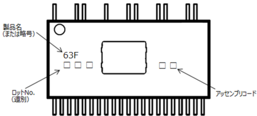
図 5.2 マーキング
