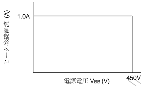
図 11.1 T_j=135^{\circ}\text{C} の安全動作領域
