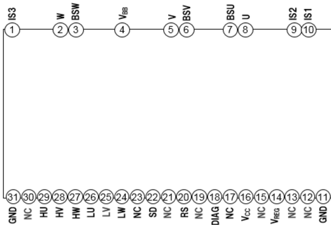
図 5.1 端子配置図
