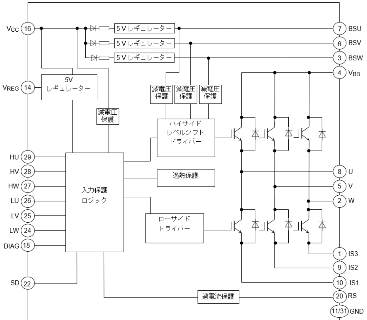
図 4.1 ブロック図
