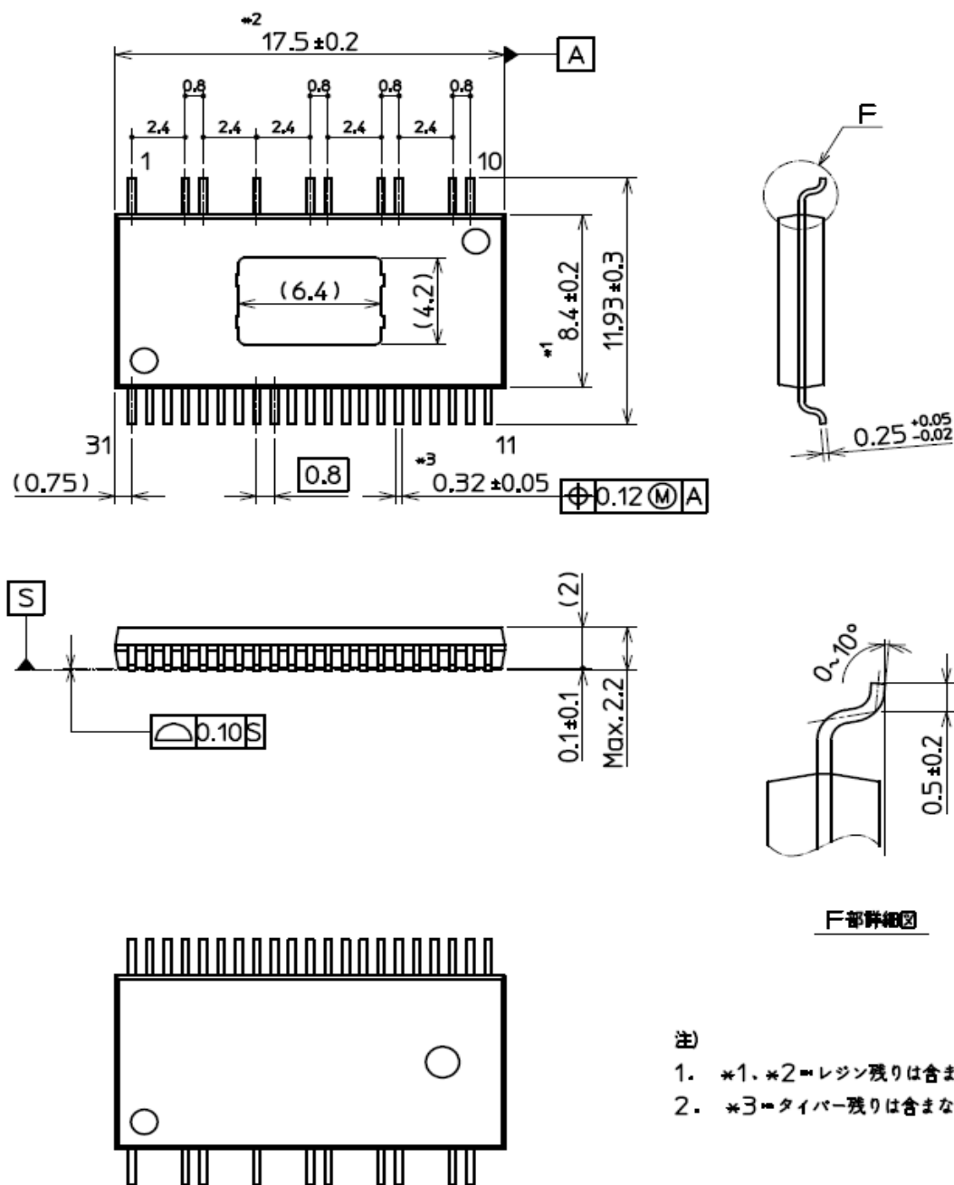
図 12.1 外形寸法図
