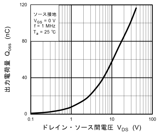
図 8.12 Q_{oss} - V_{DS}
