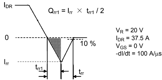
図 6.4.1 逆回復特性の測定波形図
