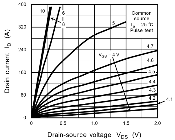
Fig. 8.2 I_D - V_{DS}
