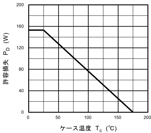
図 8.18 P_D - T_c (最大値 (保証値))
