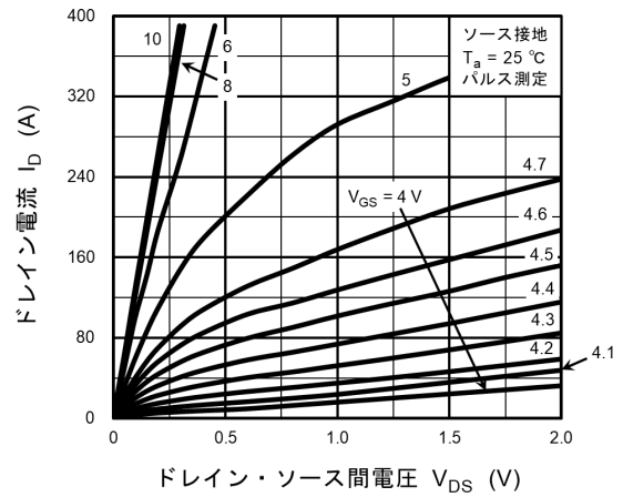
図 8.2 I_D - V_{DS}
