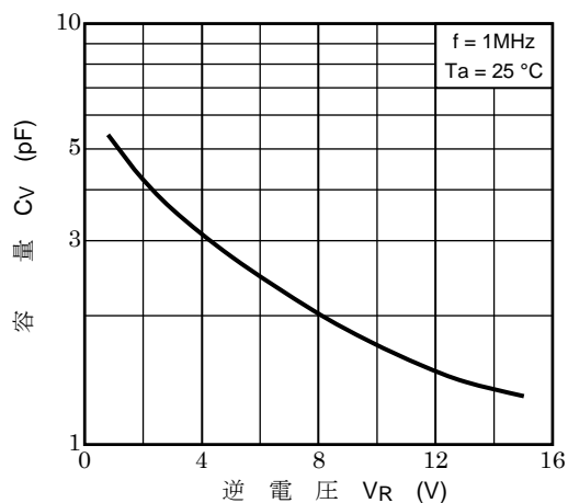
図 5-2 C_V - V_R
