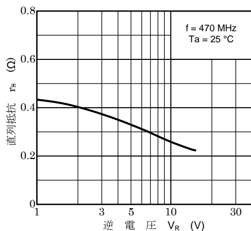
図 5-3 r_s - V_R
