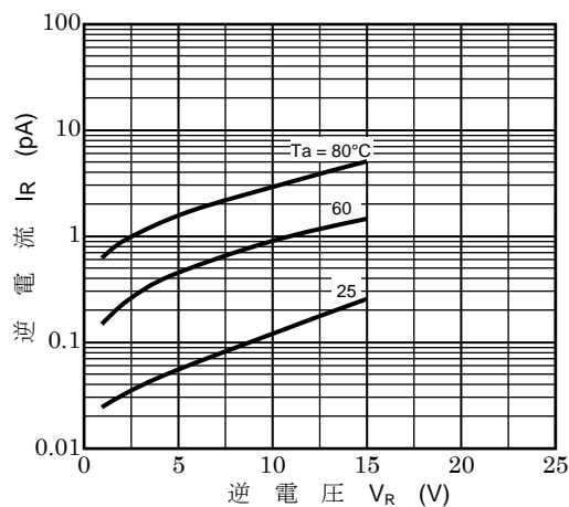
図 5-1 I_R - V_R
