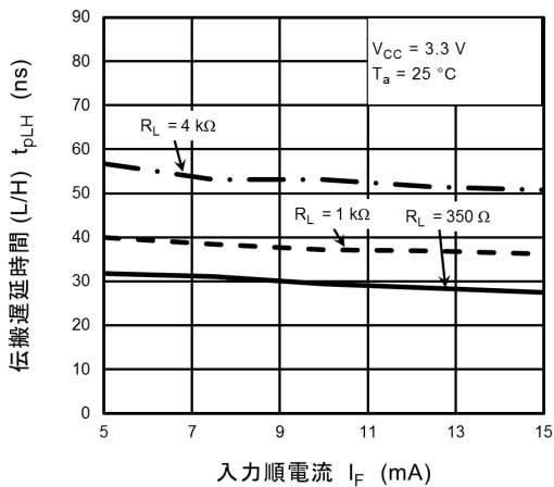
図 12.2.23 t_{pLH} - I_F
