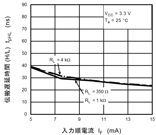
図 12.2.22 t_{pHL} - I_F
