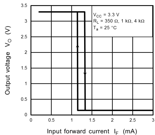
Fig. 12.2.6 V_O - I_F
