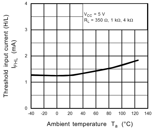
Fig. 12.2.7 I_{FHL} - T_a
