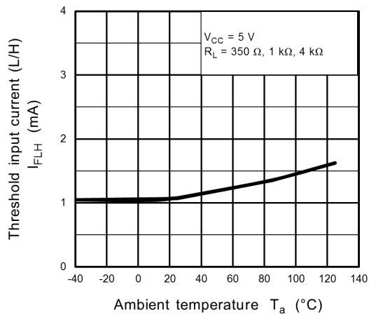
Fig. 12.2.9 I_{FLH} - T_a
