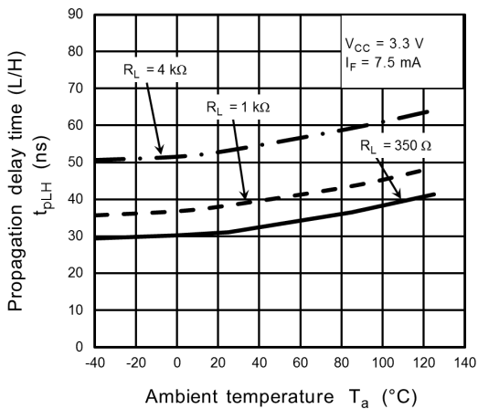
Fig. 12.2.17 t_{pLH} - T_a
