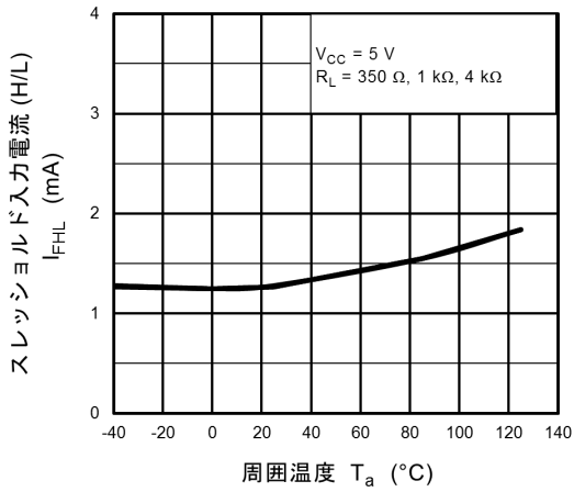
図 12.2.7 I_{FHL} - T_a
