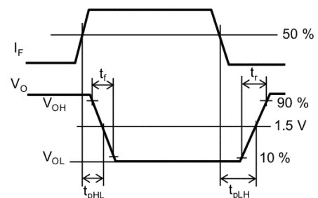
図 12.1.6 伝搬遅延時間測定回路, 波形
