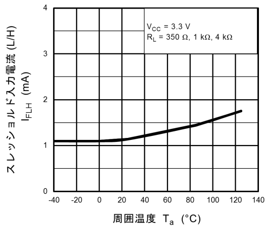
図 12.2.10 I_{FLH} - T_a
