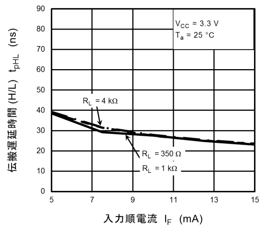
図 12.2.22 t_{pHL} - I_F
