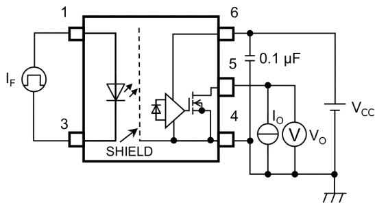
図 12.1.5 I_{FHL} , I_{FLH} , I_{HYS} 測定回路
