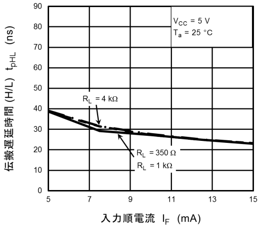
図 12.2.19 t_{pHL} - I_F
