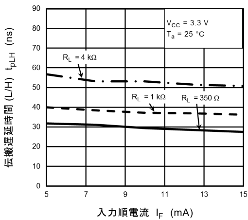
図 12.2.23 t_{pLH} - I_F
