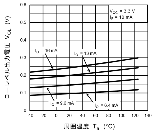
図 12.2.4 V_{OL} - T_a
