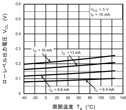
図 12.2.3 V_{OL} - T_a
