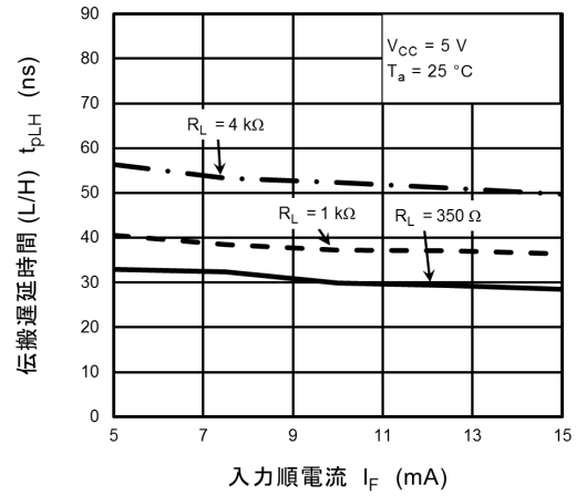
図 12.2.20 t_{pLH} - I_F
