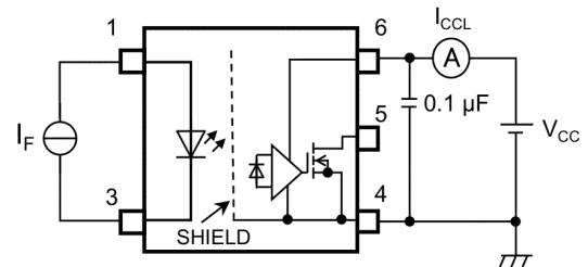
図 12.1.4 I_{CCL} 測定回路
