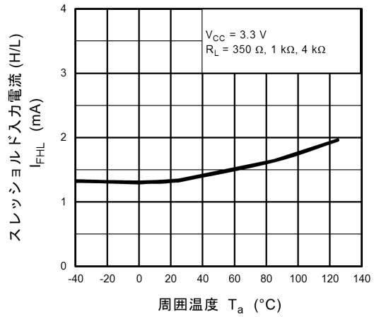
図 12.2.8 I_{FHL} - T_a
