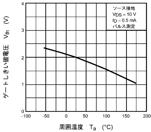
図 8.9 V_{th} - T_a
