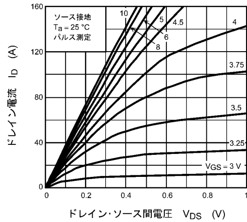
図 8.2 I_D - V_{DS}
