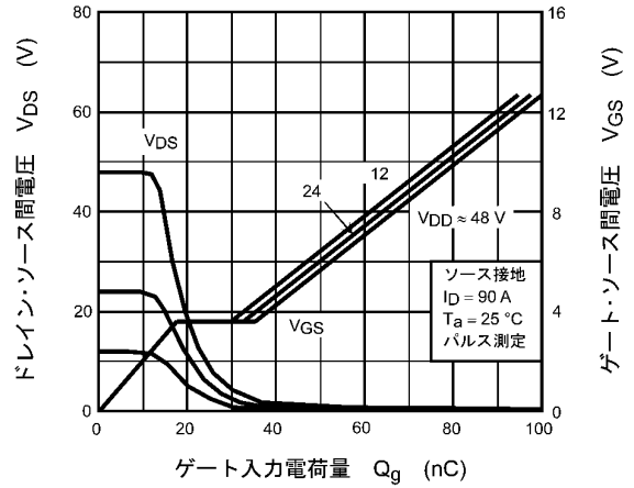
図 8.10 ダイナミック入出力特性
