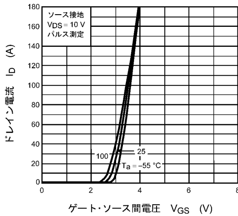
図 8.3 I_D - V_{GS}
