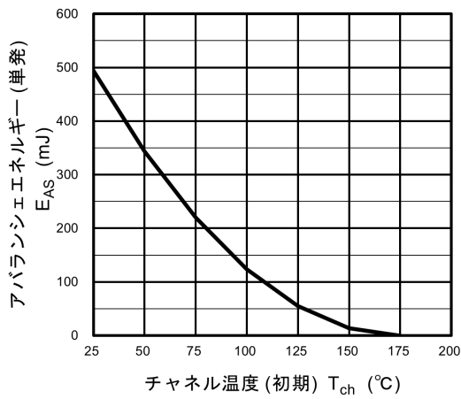
図 8.15 E_{AS} - T_{ch} (最大値 (保証値))
