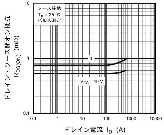
図 8.8 R_{DS(ON)} - I_D
