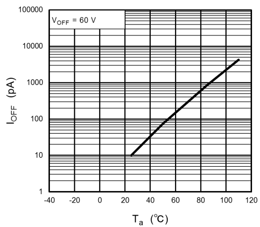
図 12.10 I_{OFF} - T_a
