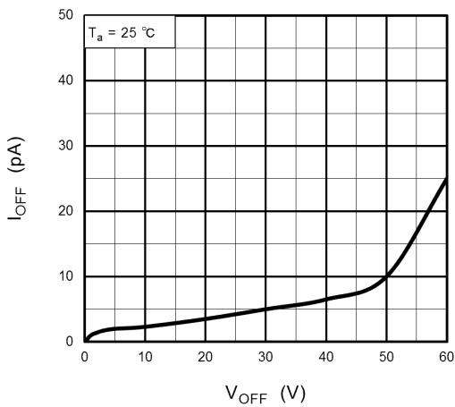
図 12.9 I_{OFF} - V_{OFF}
