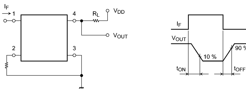
図 11.1 スイッチング時間測定回路
