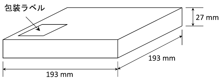
図 16.4.1 1リール入り梱包箱
