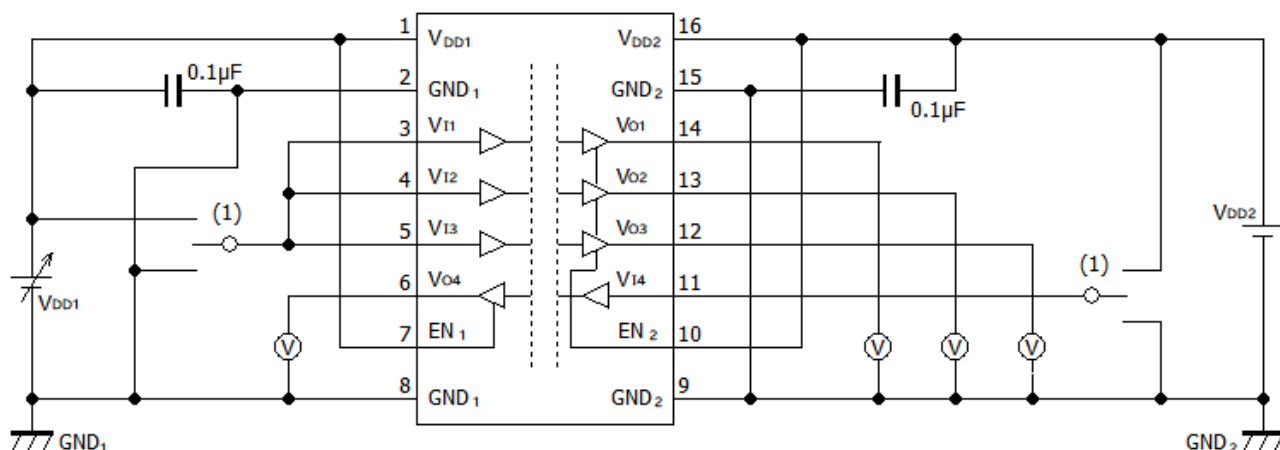
図 12-1 : DCL541L01/DCL541H01 V_{DD1UV+}/V_{DD1UV-} 特性測定回路図
