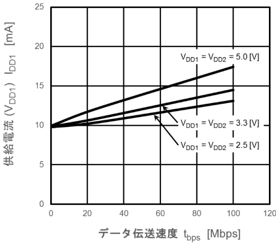
図 13.1 : DCL541x01 I DD1 動作電流 - データレート
