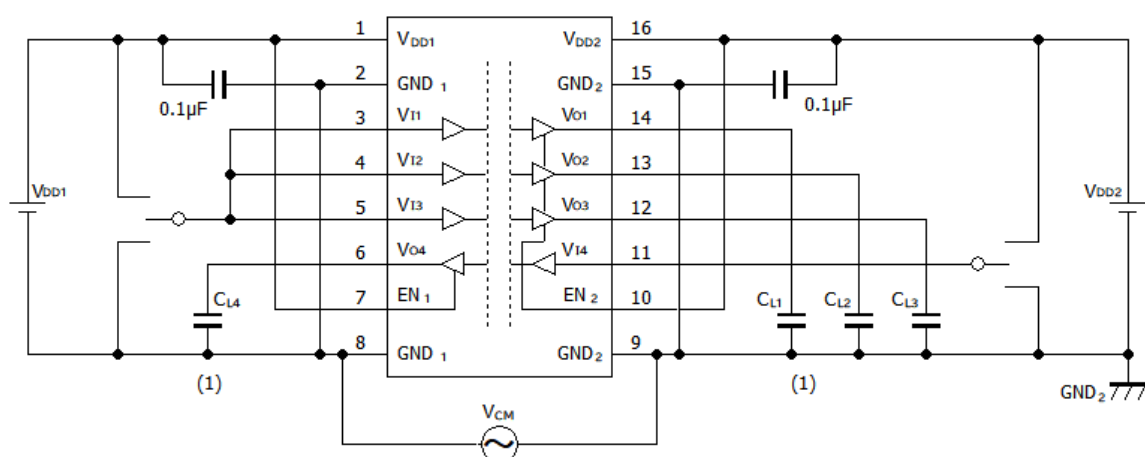
図 12-15 : DCL541L01/DCL541H01 コモンモード過渡耐性テスト回路図
