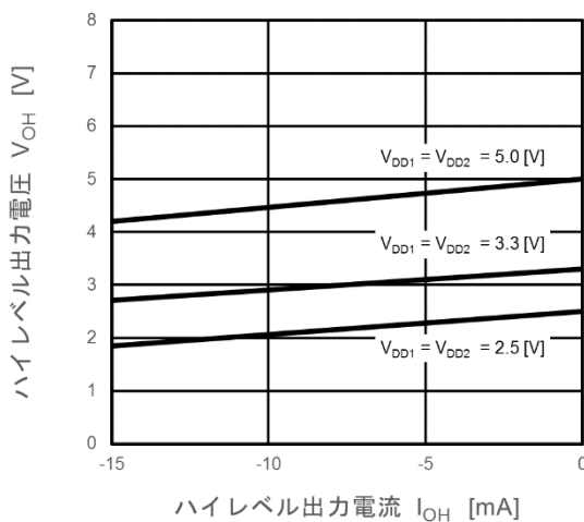
図 13-5 : V_{OH} - I_{OH}
