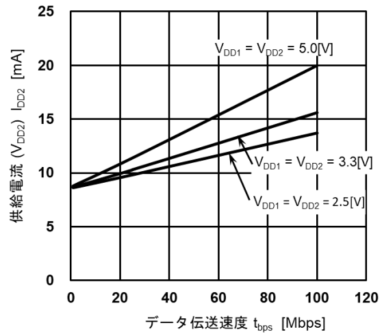
図 13.4 : DCL542x01 I DD2 動作電流 - データレート
