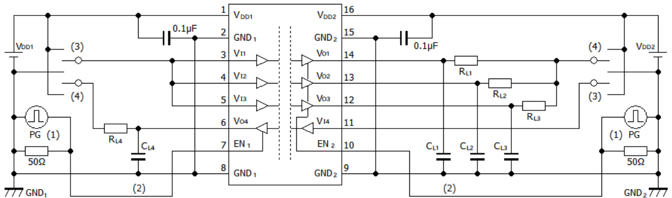
図 12-12 : DCL541L01/ DCL541H01 イネーブル伝搬遅延時間テスト回路図
