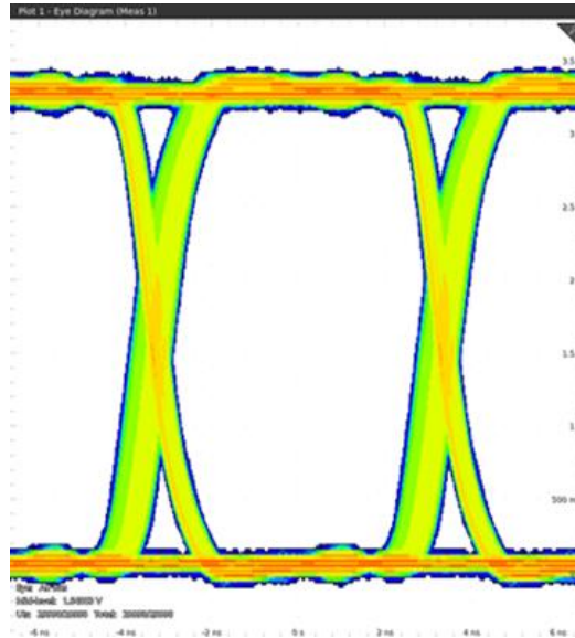
図 14-1 : DCL541L01 のアイ・ダイアグラム例
