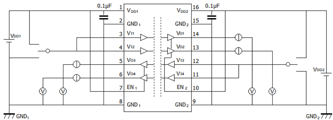
图 12.6 : DCL542L01/DCL542H01 V_{OH}/V_{OL} 特性測定回路図
