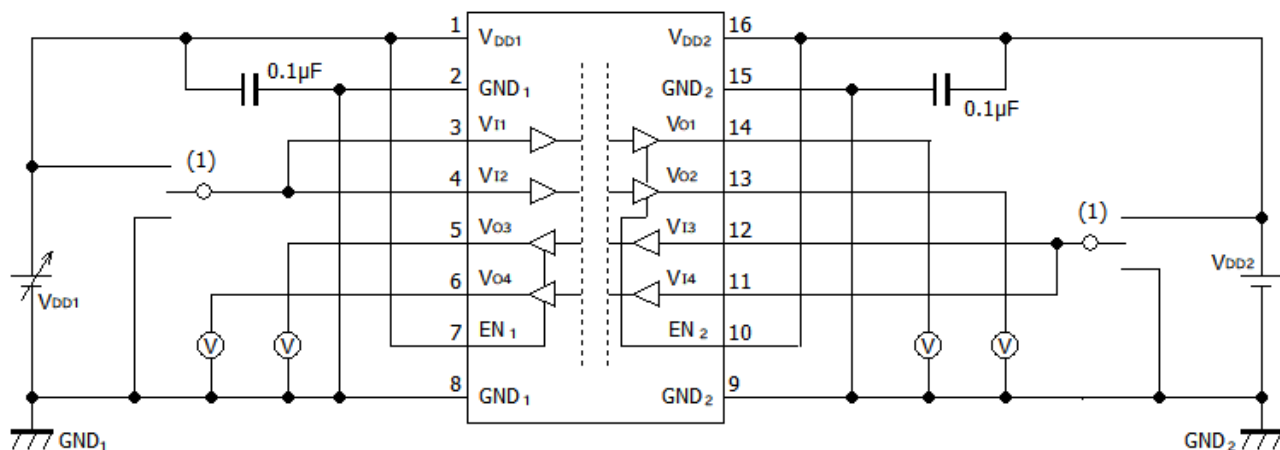
図 12-2 : DCL542L01/DCL542H01 V_{DD1UV+}/V_{DD1UV-} 特性測定回路図
