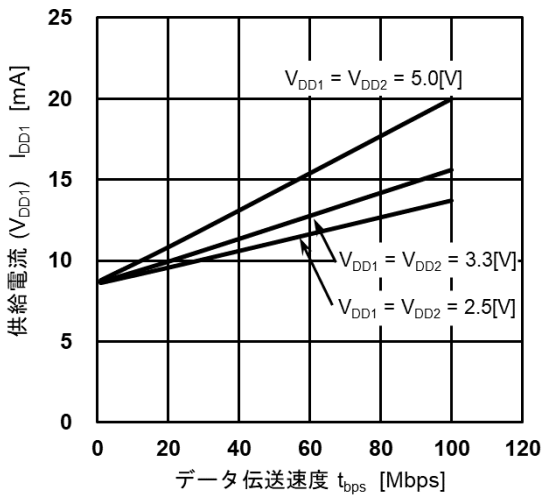
図 13.3 : DCL542x01 I DD1 動作電流 - データレート
