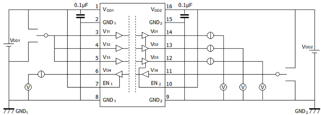
图 12.5 : DCL541L01/DCL541H01 V_{OH}/V_{OL} 特性測定回路図
