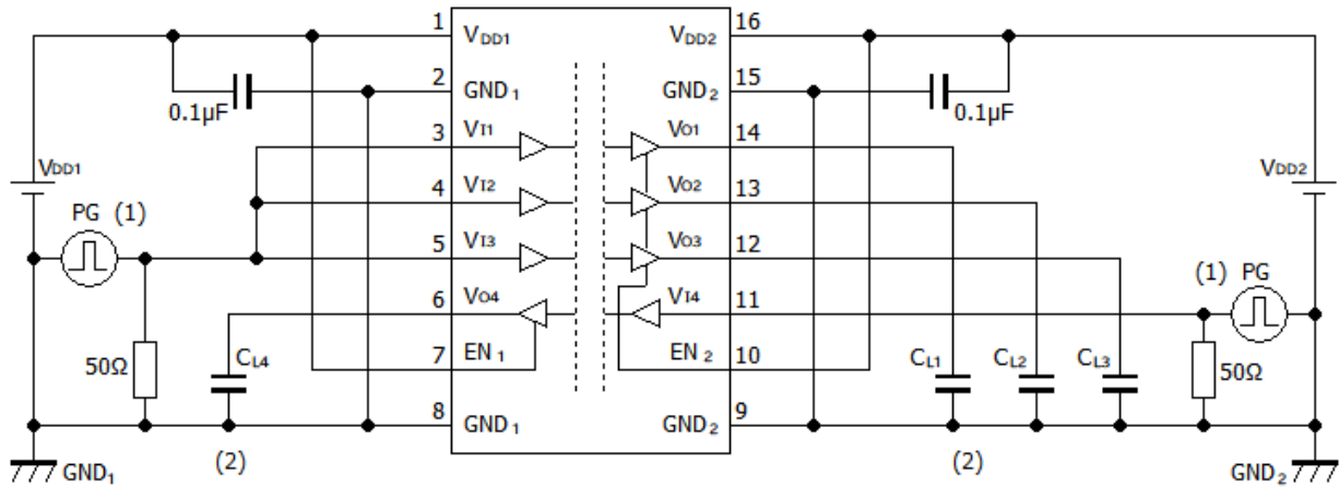
図 12-9 : DCL541L01/DCL541H01 Switching 特性測定回路図
