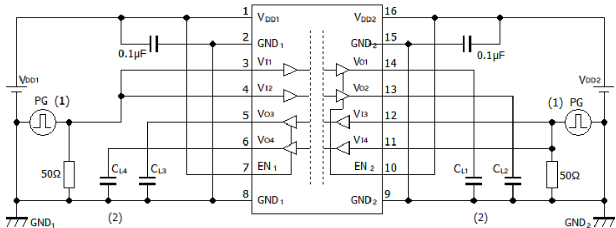
図 12-10 : DCL542L01/DCL542H01 Switching 特性測定回路図
