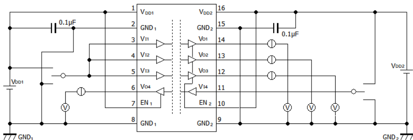
图 12-5 : DCL541L01/DCL541H01 V_{OH}/V_{OL} 特性测定回路图
