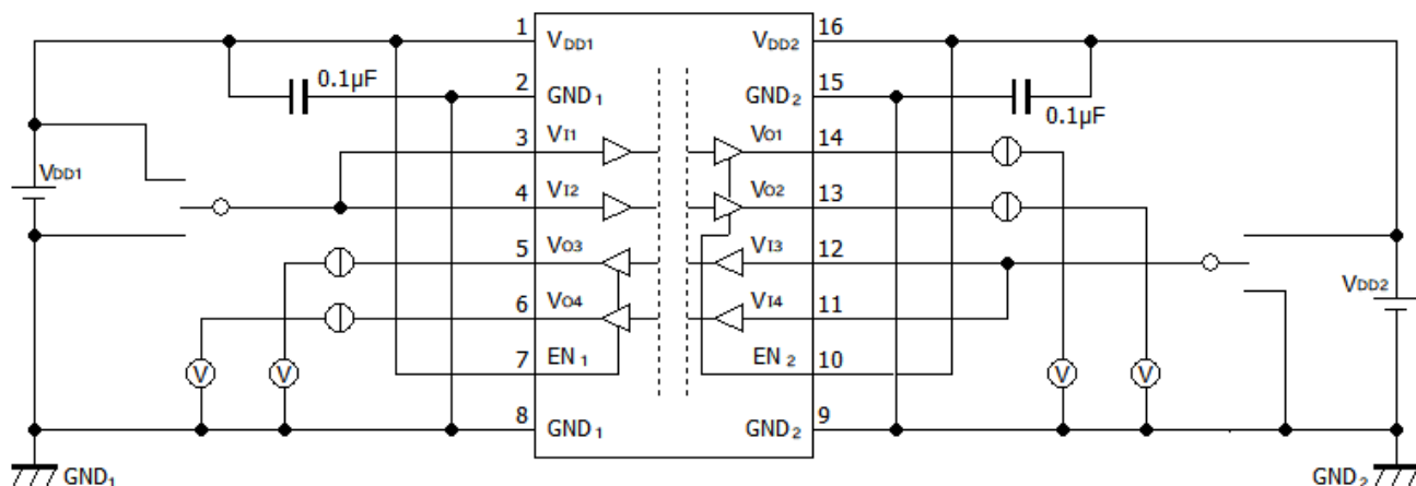
图 12-6 : DCL542L01/DCL542H01 V_{OH}/V_{OL} 特性测定回路图
