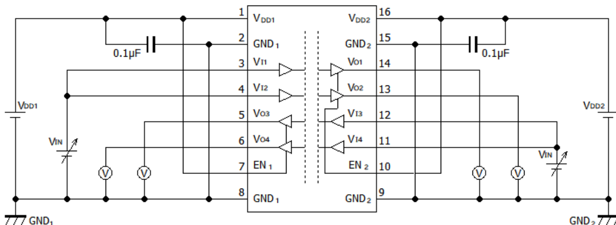
图 12-8 : DCL542L01/DCL542H01 V_{IH}/V_{IL} 特性测定回路图
