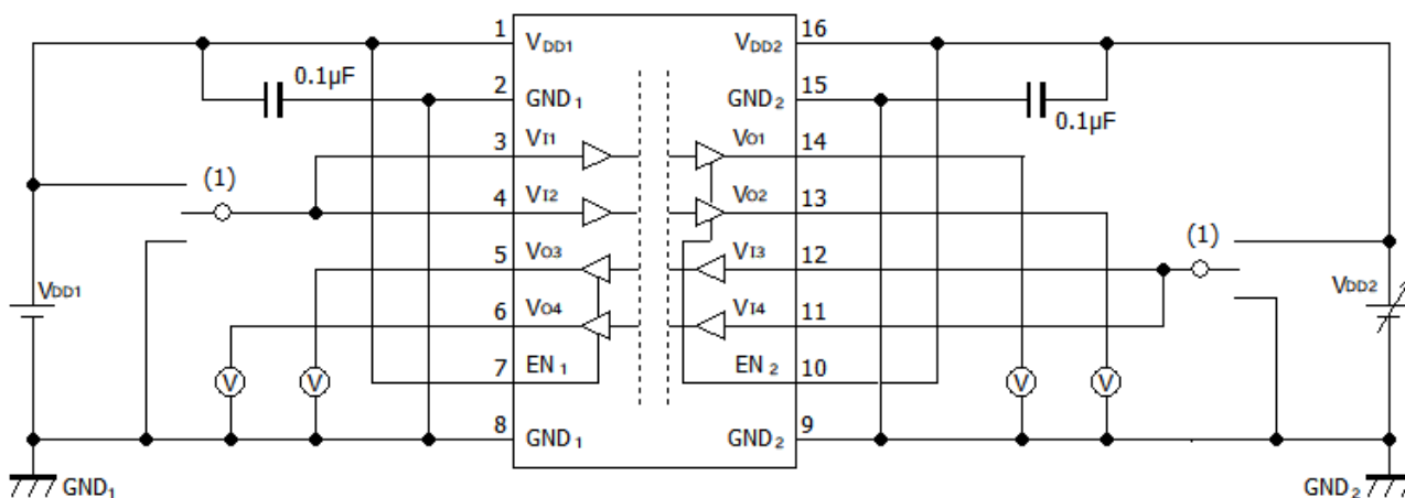
图 12-4 : DCL542L01/DCL542H01 V_{DD2UV+}/V_{DD2UV-} 特性測定回路図
