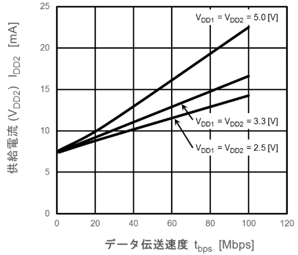
図 13.2 : DCL541x01 I DD2 動作電流 - データレート
