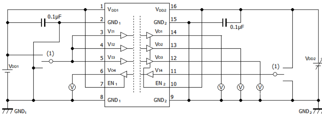
图 12-3 : DCL541L01/DCL541H01 V_{DD2UV+}/V_{DD2UV-} 特性測定回路図
