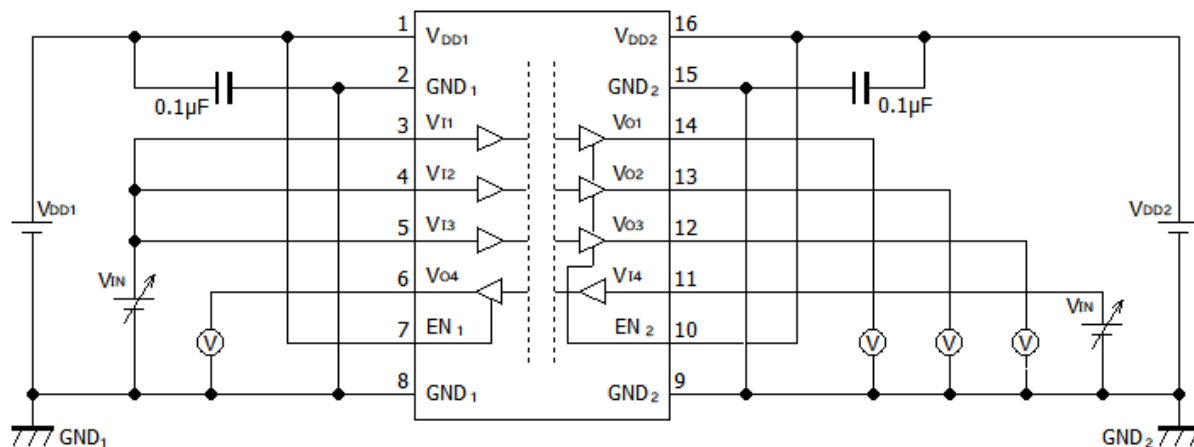
图 12-7 : DCL541L01/DCL541H01 V_{IH}/V_{IL} 特性测定回路图
