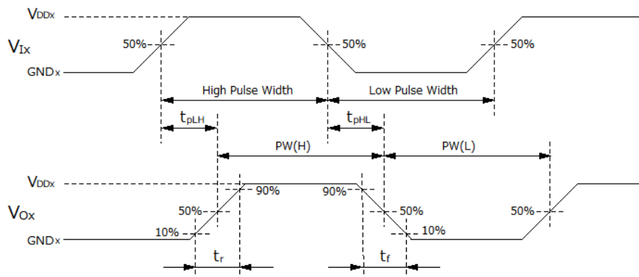
図 12-11 : Switching 特性波形図
