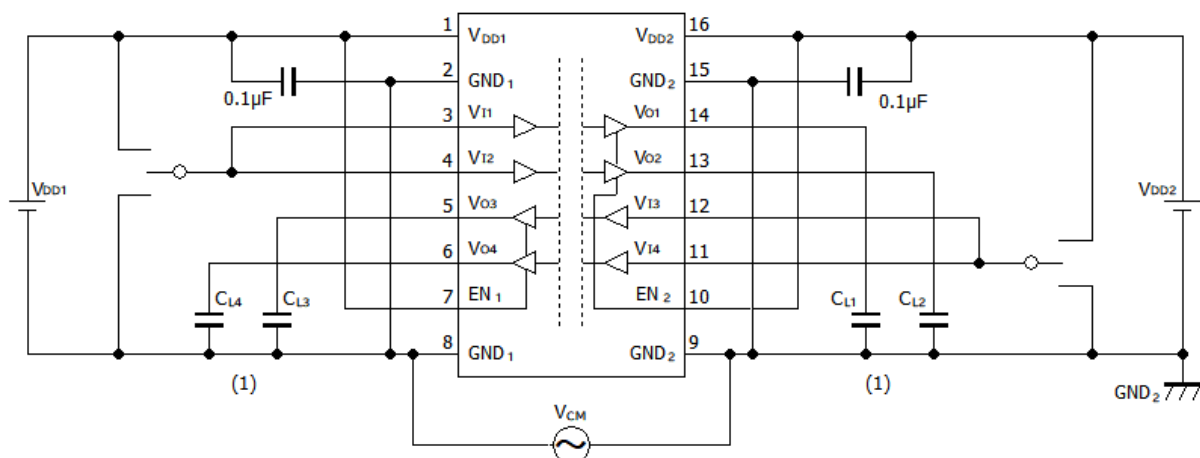
図 12-16 : DCL542L01/DCL542H01 コモンモード過渡耐性テスト回路図
