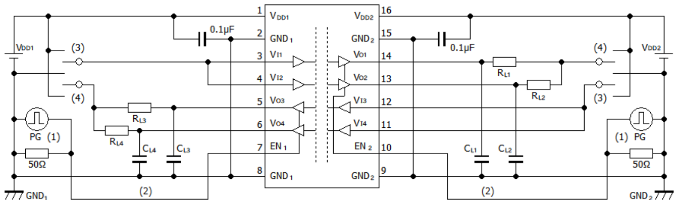
図 12-13 : DCL542L01/ DCL542H01 イネーブル伝搬遅延時間テスト回路図
