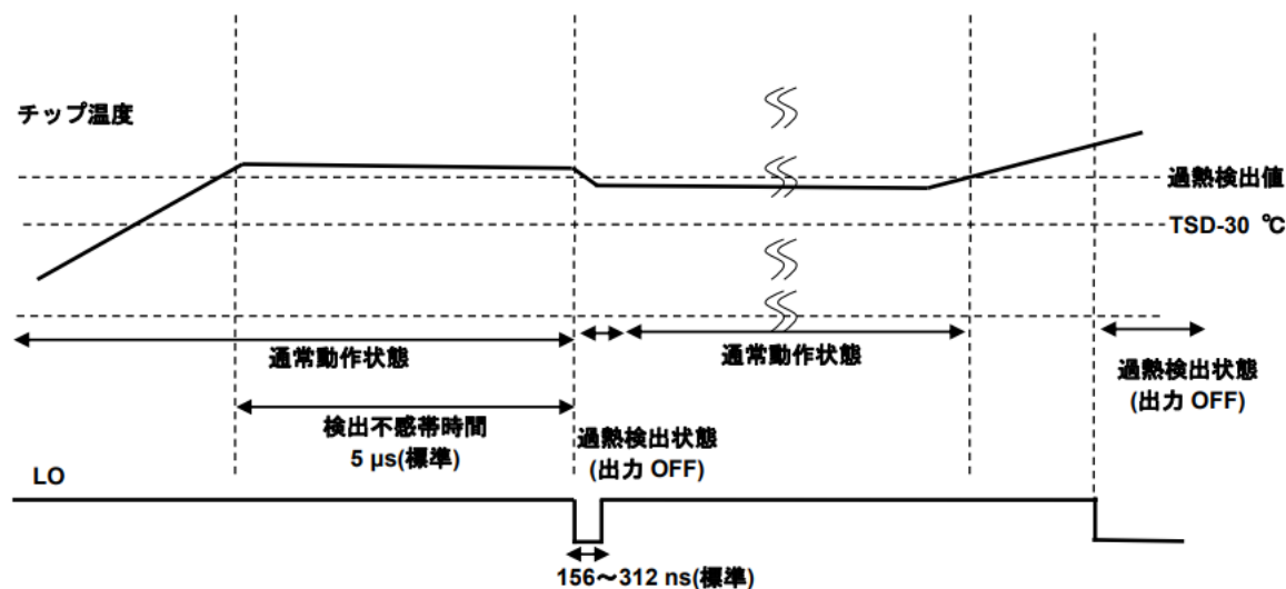
図 5.2 過熱検出のタイミングチャート 2
