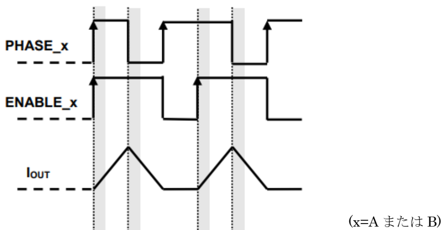
図 4.3 入力信号と tBLK の不感帯時間タイミングチャート
