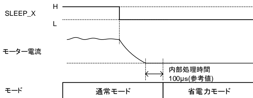
図 3.1 SLEEP_X タイミング
