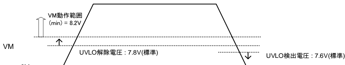
図 1.1 VM 動作範囲と UVLO しきい値
