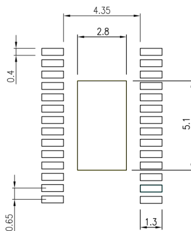
図 8.1 参考ランドパターン
