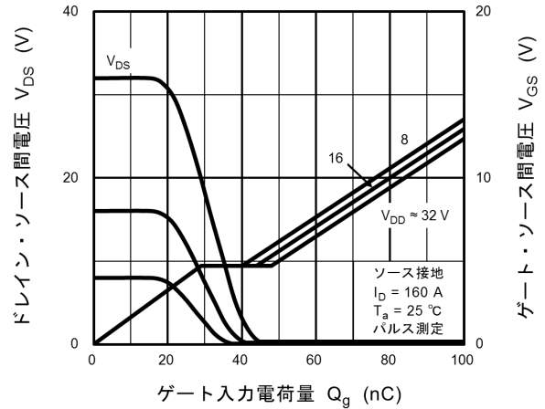
ゲート入力電荷量 Q_g (nC) 図 8.14 ダイナミック入出力特性
