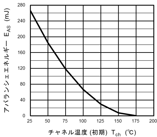
チャンネル温度 (初期) T_{ch} (°C) 図 8.15 E_{AS} - T_{ch} (最大値 (保証値))
