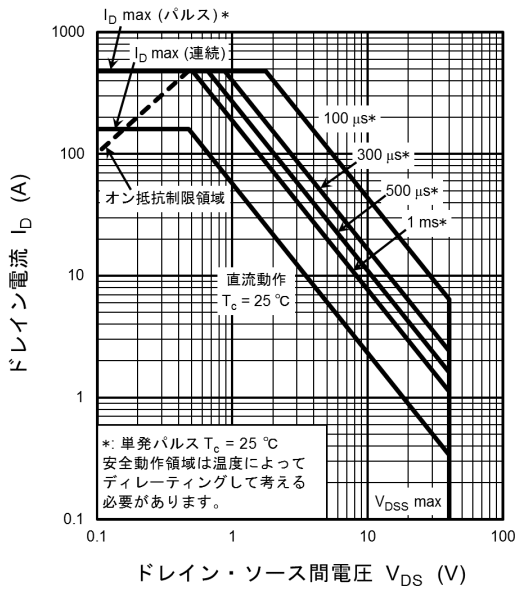
図 8.18 安全動作領域 (最大値 (保証値))
