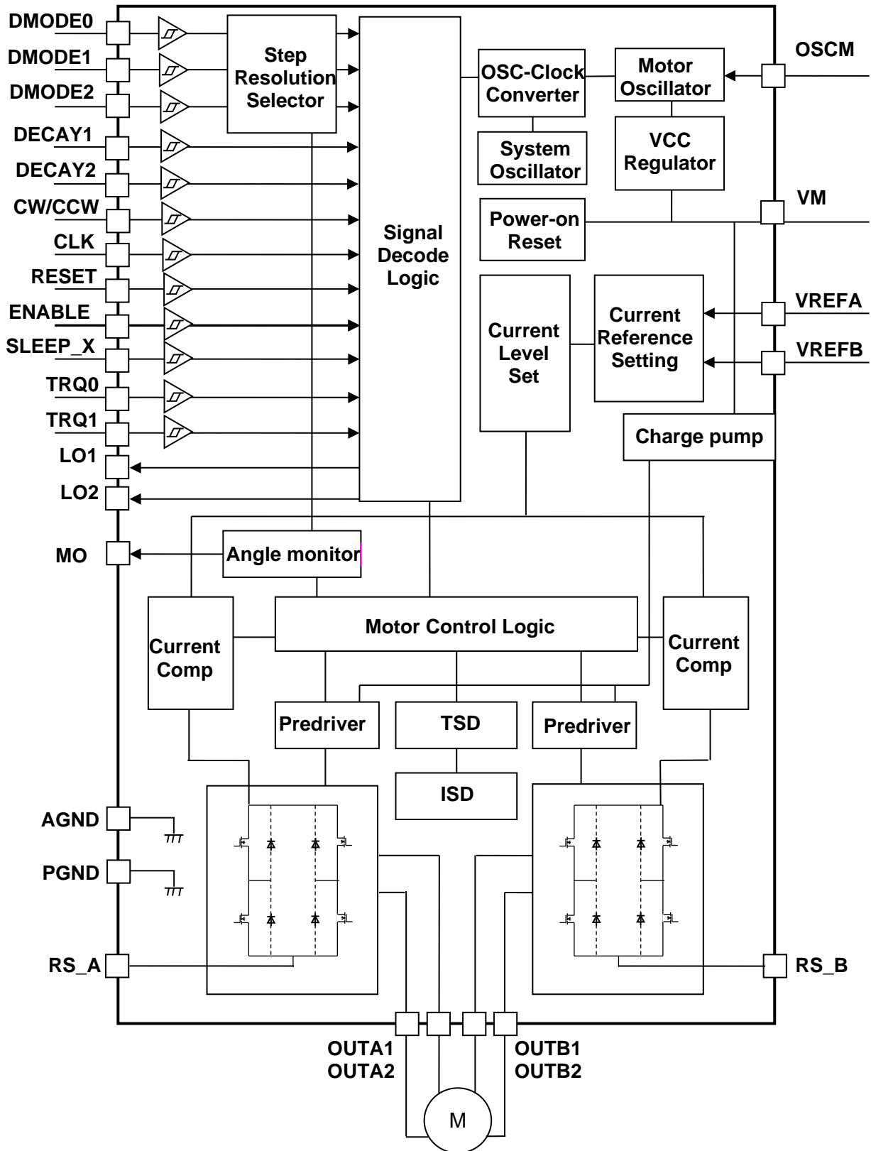
図4 ブロック図
