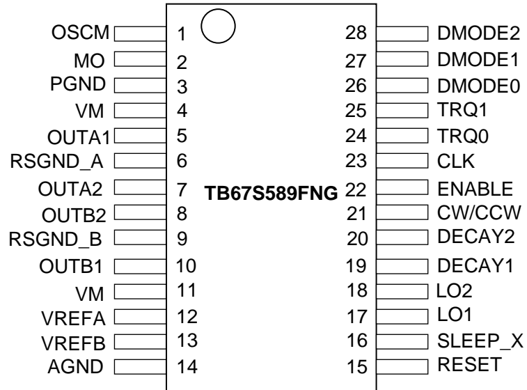
図3 ピン配置図
