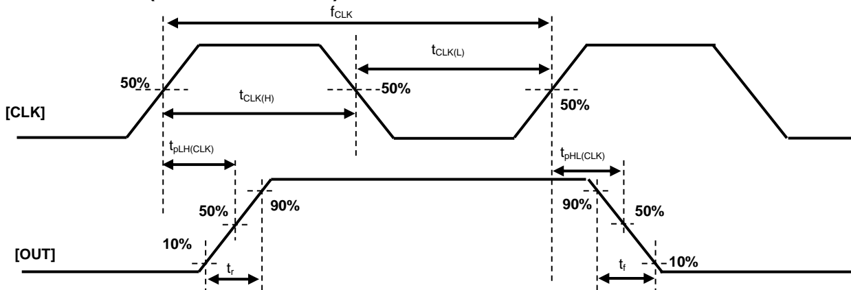
図 20.1 TB67S589FNG(CLK と出力の関係)
