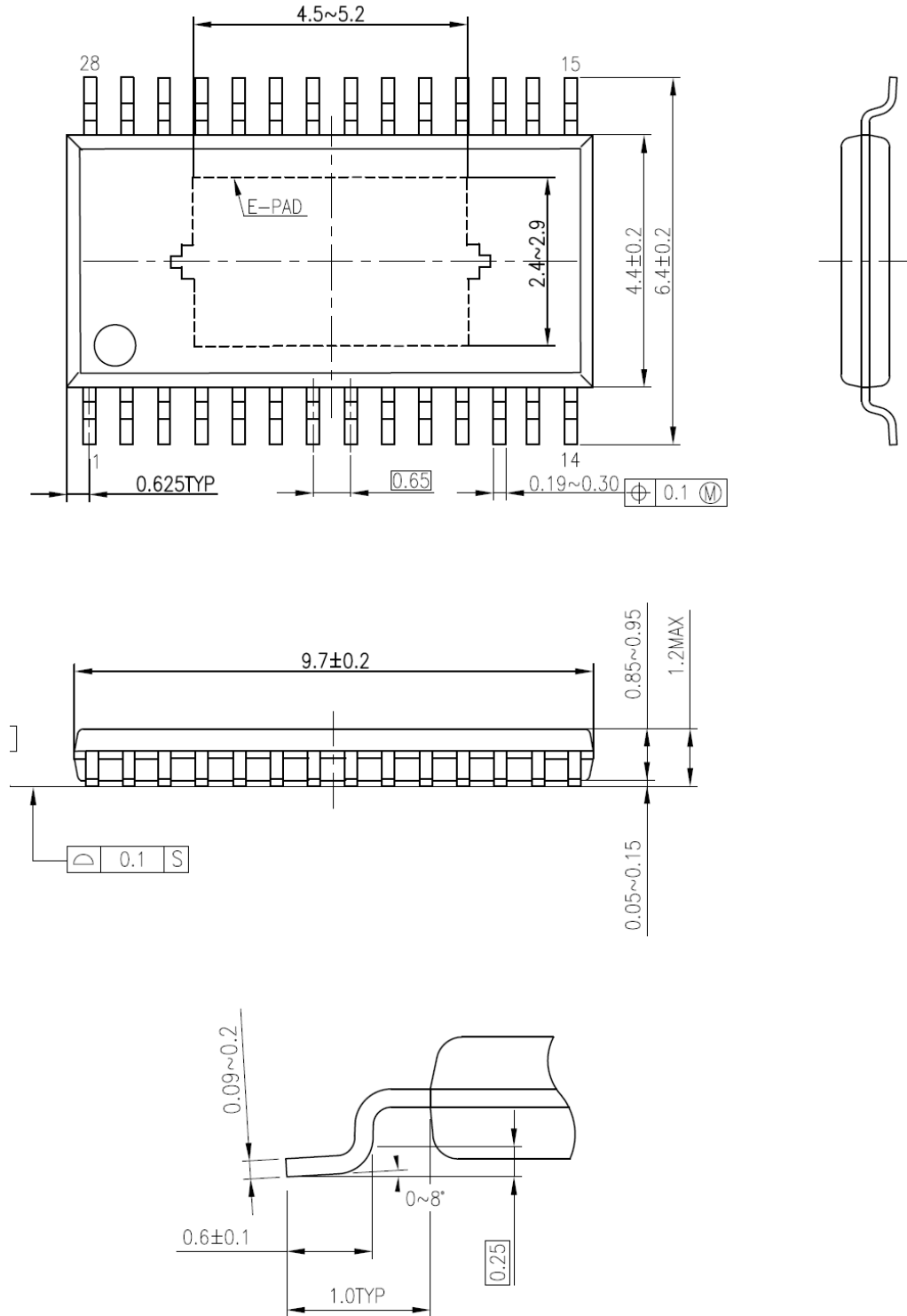
図 21 外形図
