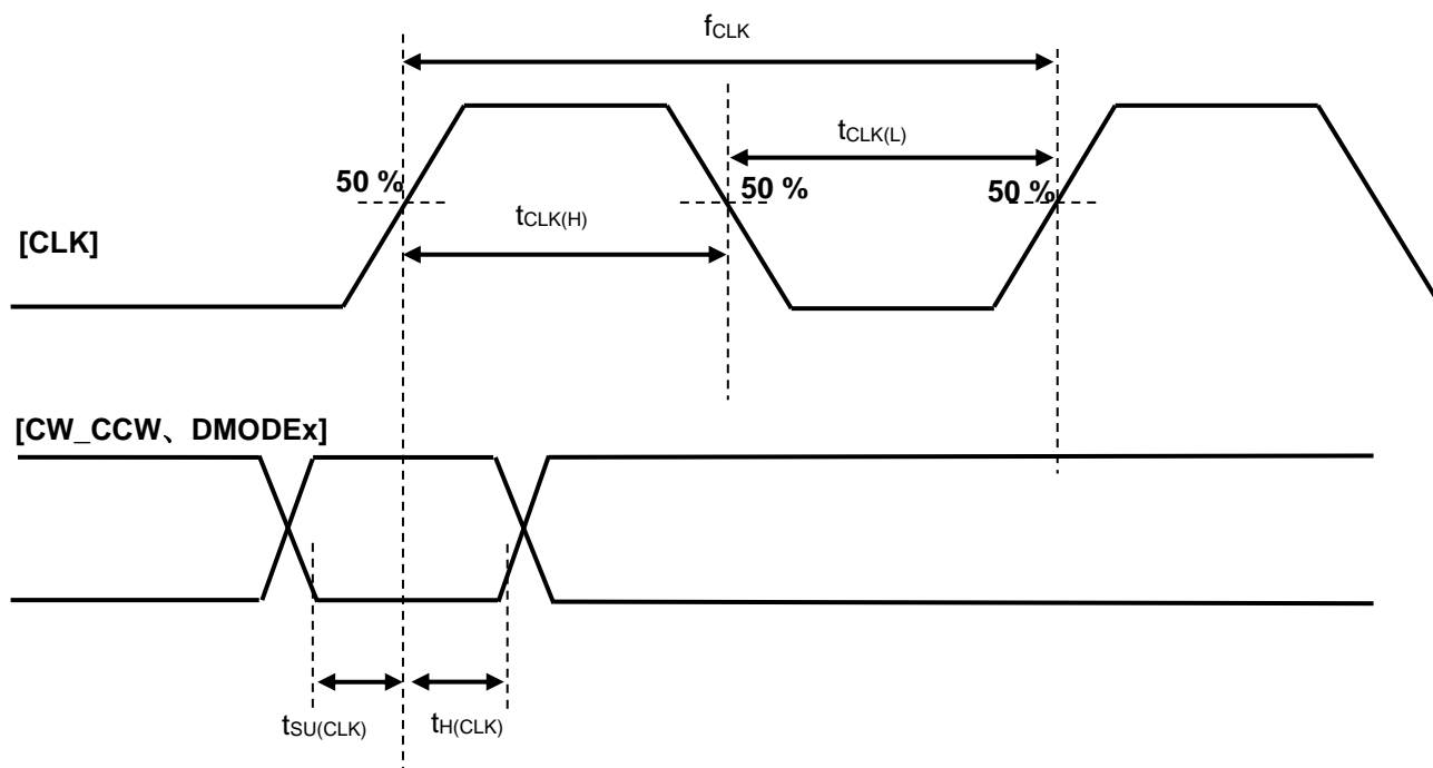
図 20.2 TB67S589FNG(CLK とその他制御信号の関係)
