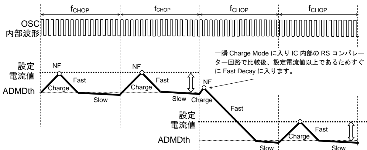
図 7.14.3 設定電流値が減少方向の場合
