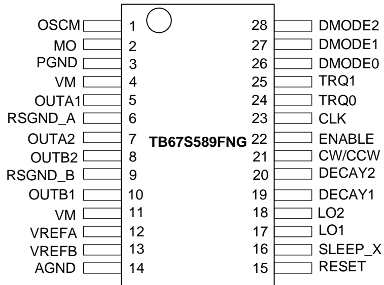
図3 ピン配置図
