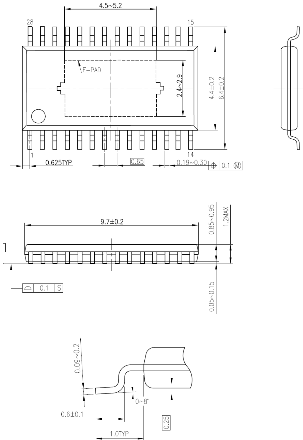
图 24 外形图
