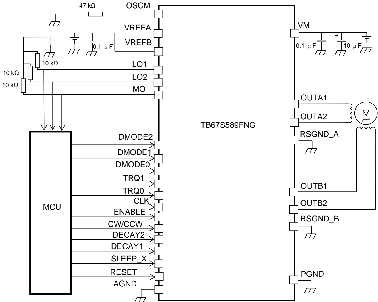
図 21 応用回路例
