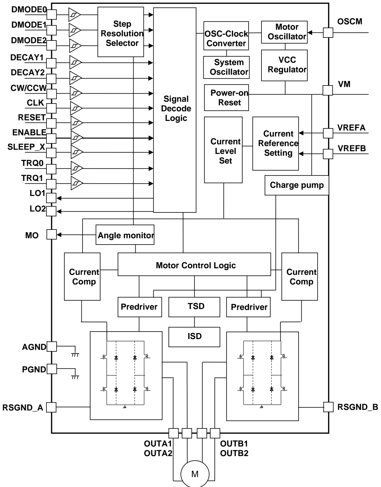
図 4 ブロック図
