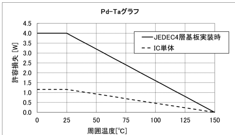
図 16 PD-Ta グラフ
