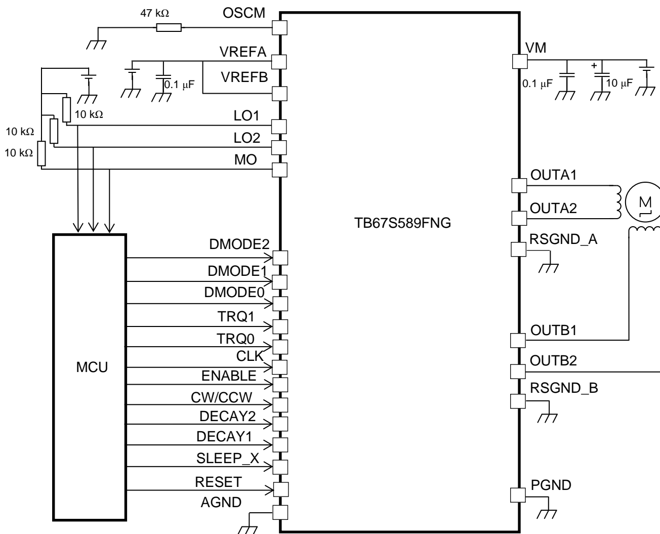
図 21 応用回路例
