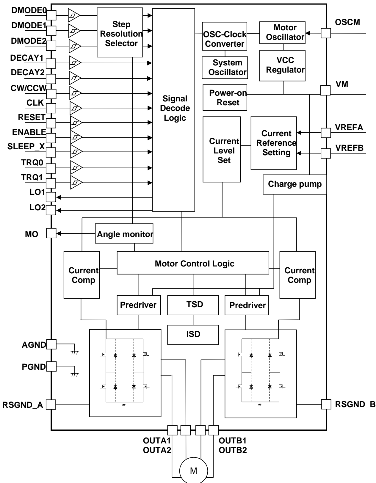
図4 ブロック図
