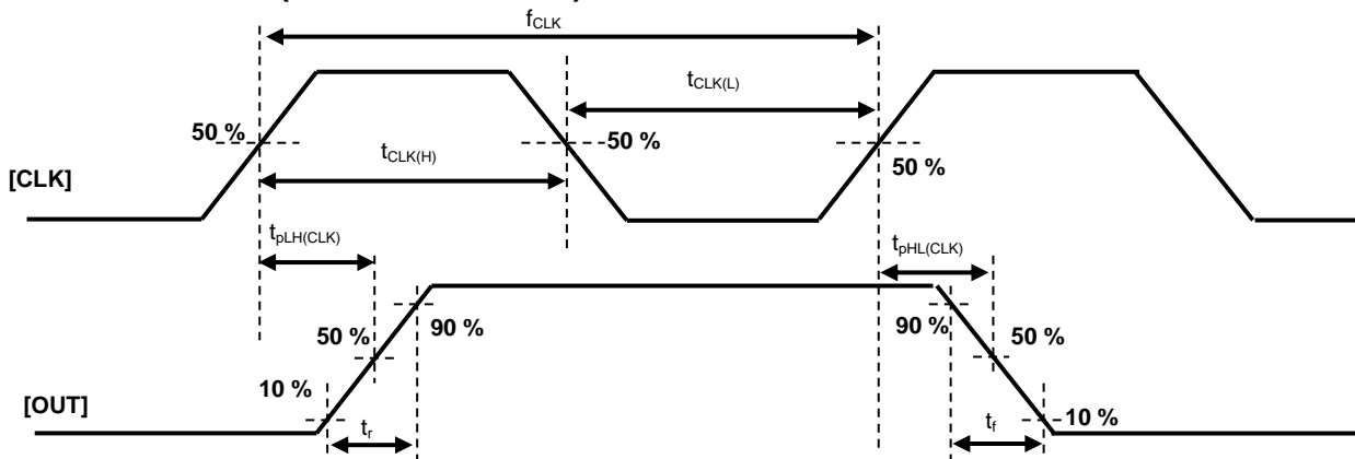
図 20.1 TB67S589FTG(CLK と出力の関係)
