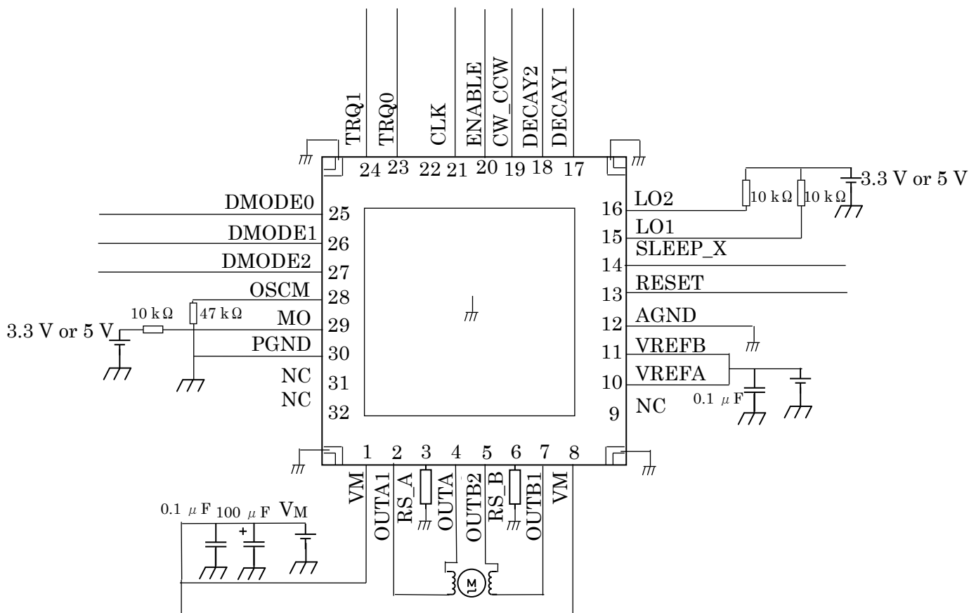
図 21 応用回路例
