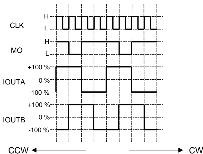
図 7.6.1 2 相励磁設定
