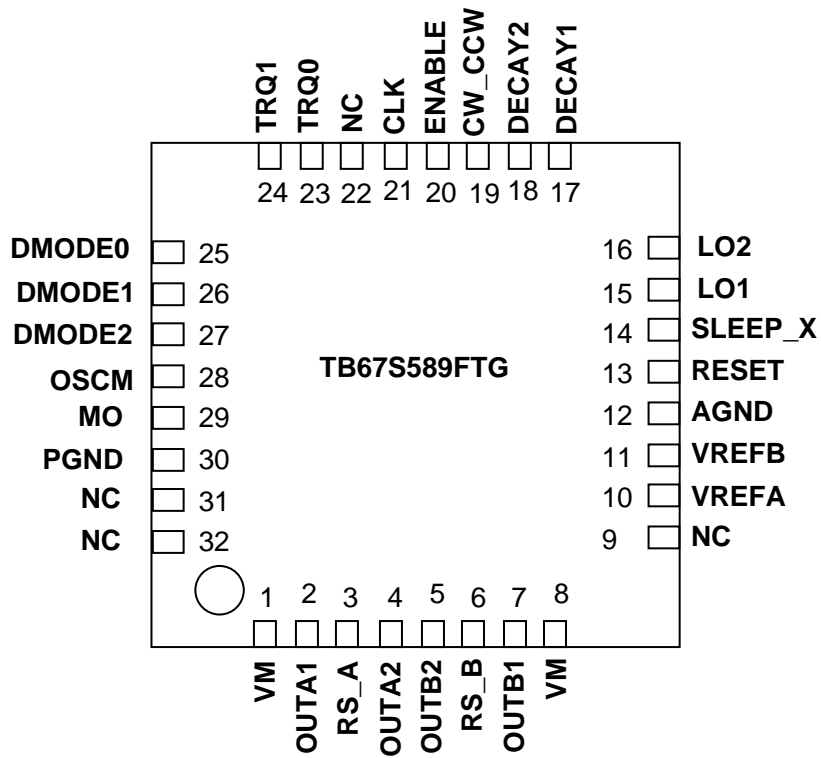
図3 ピン配置図
