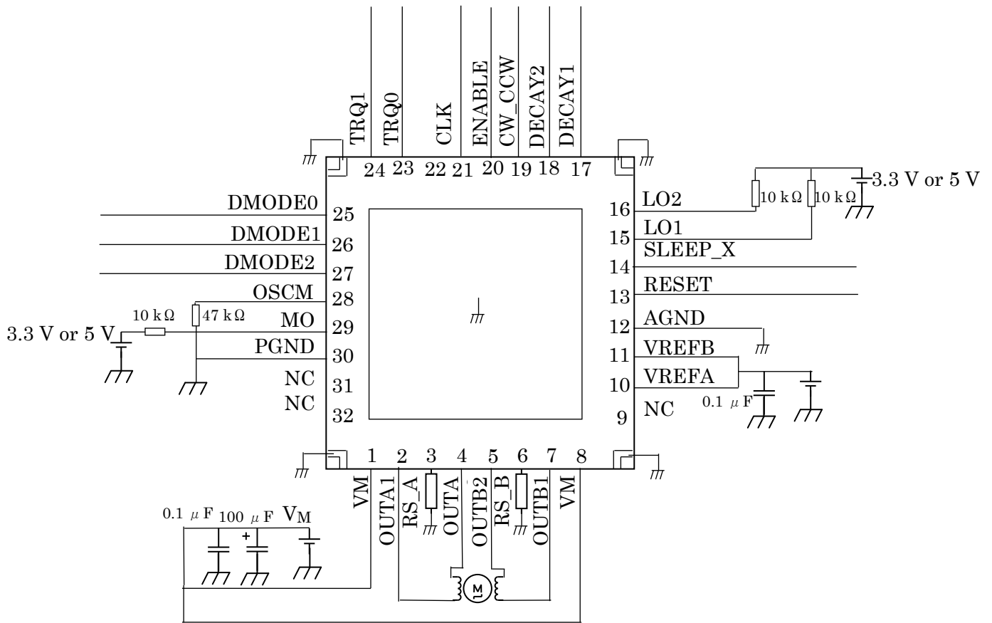
図 21 応用回路例
