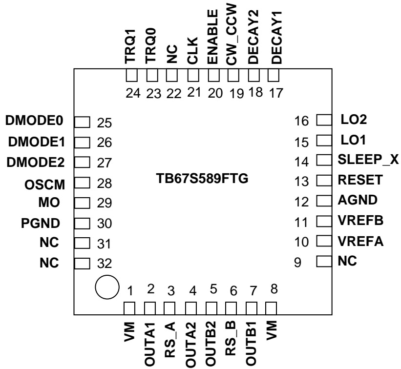
図3 ピン配置図
