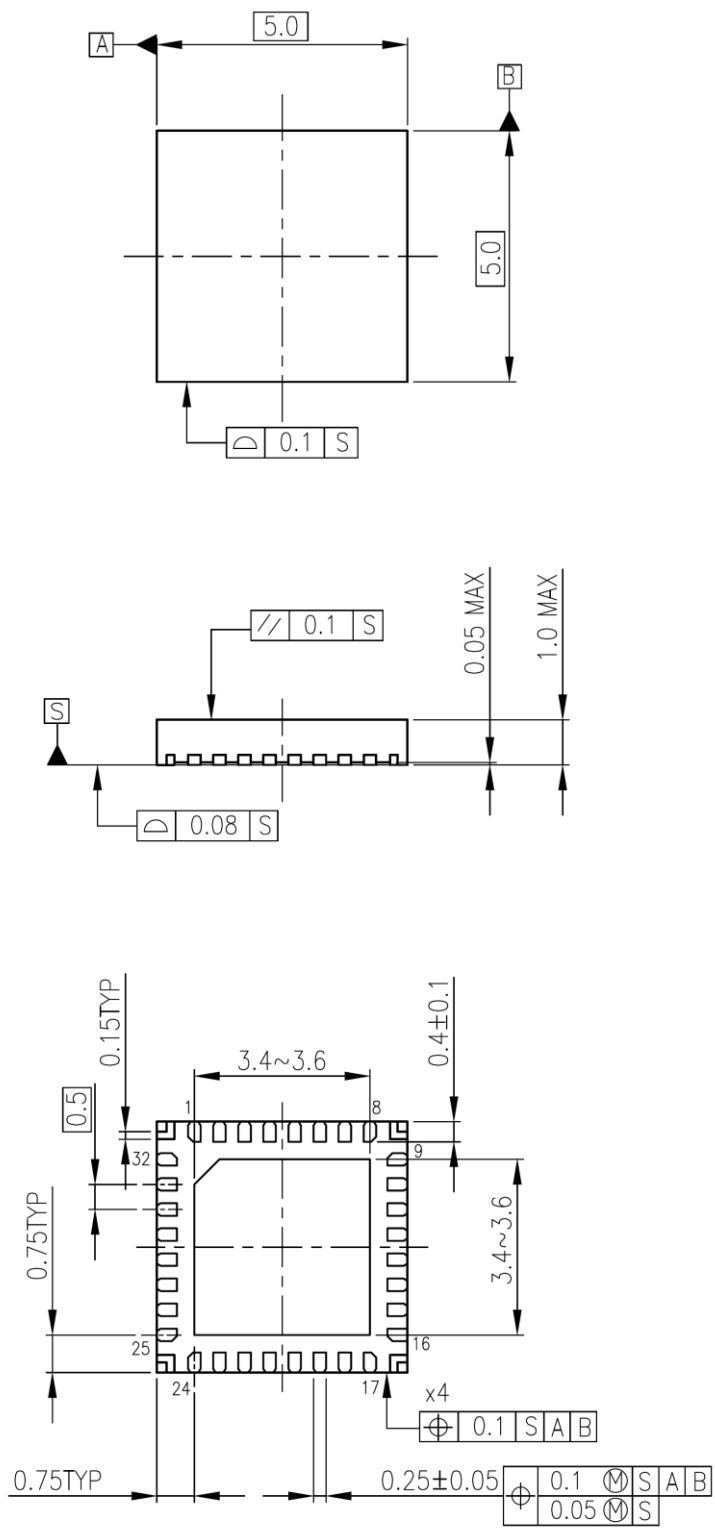
图 21 外形图
