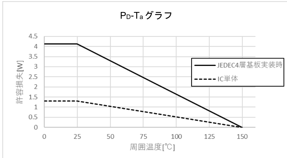
図 16 P D -T a グラフ
