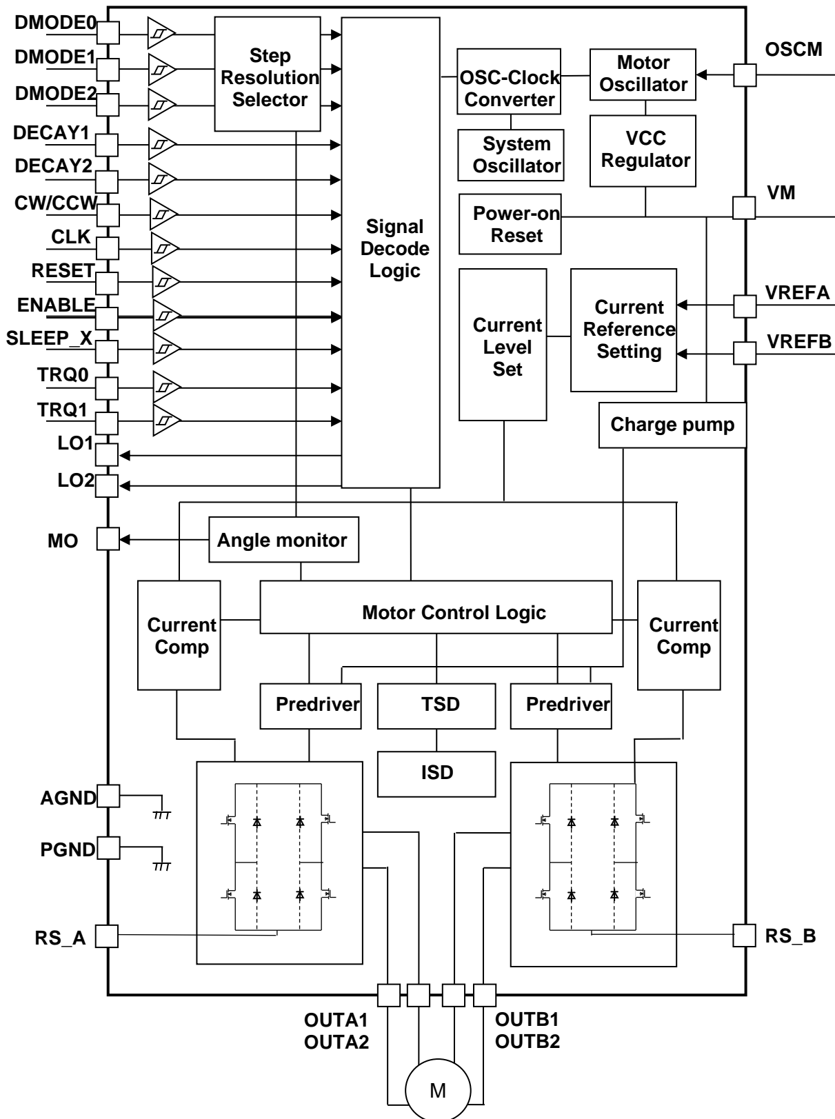
図4 ブロック図
