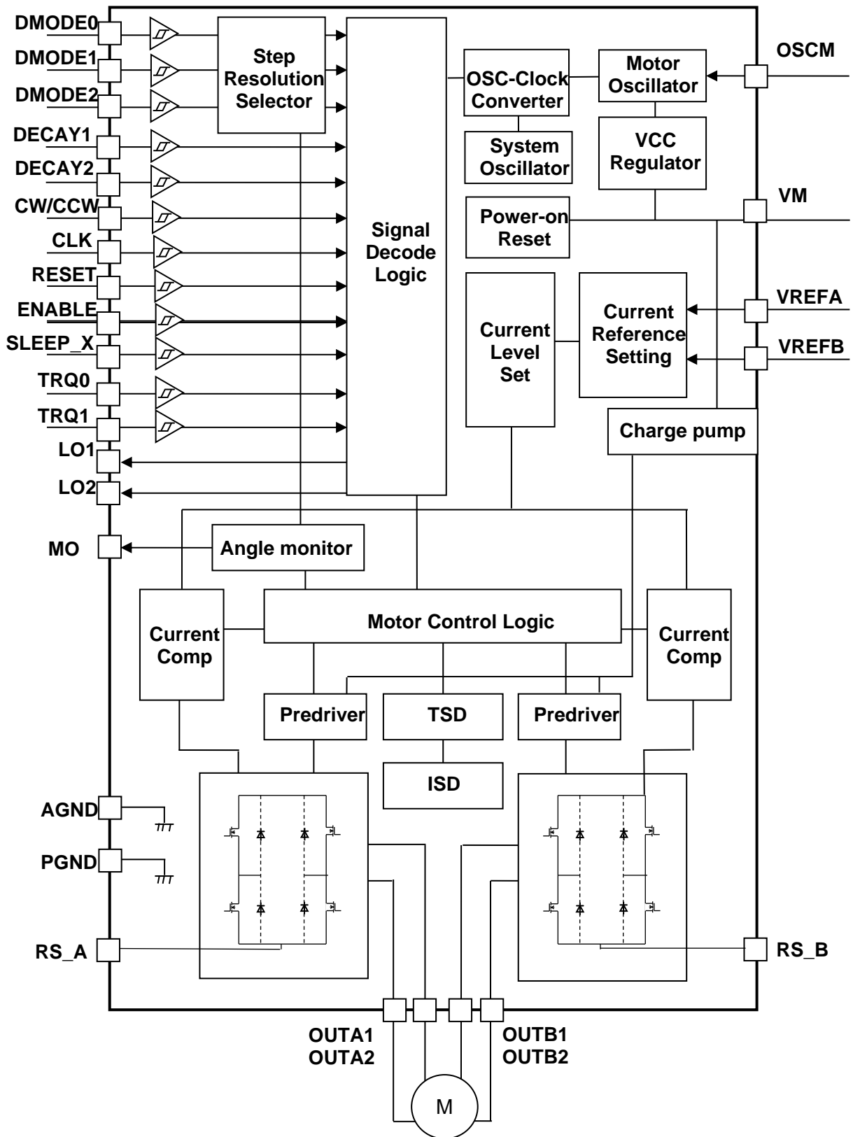
図4 ブロック図
