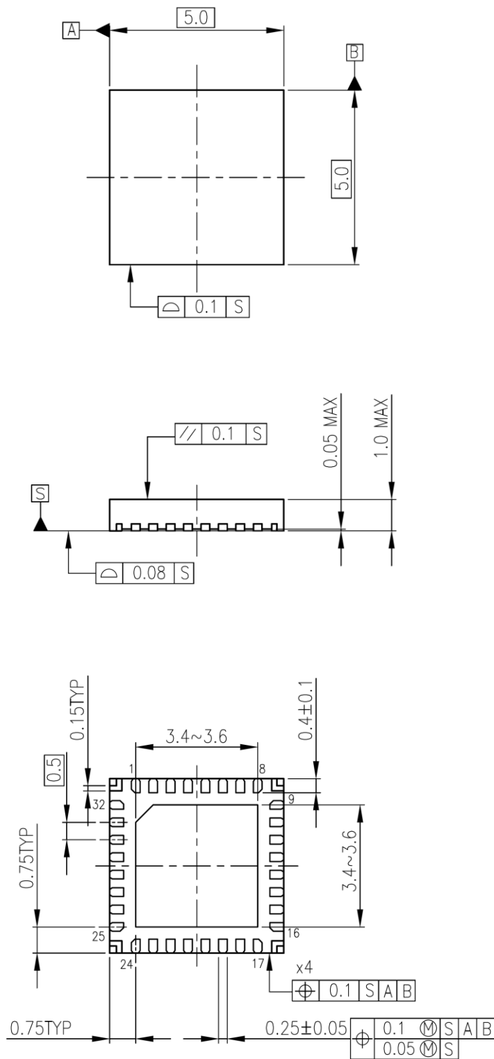
图 21 外形图
