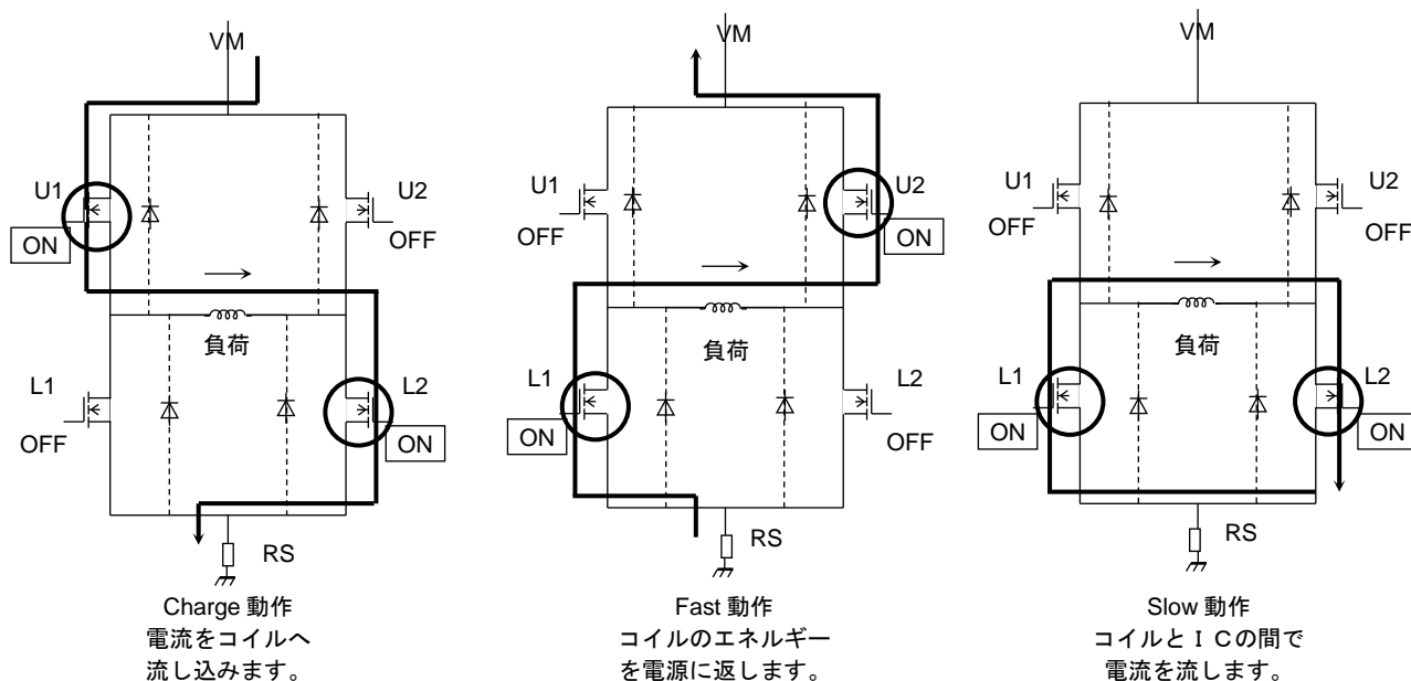
図 8 出力段トランジスタ動作モード (Advanced Dynamic Mixed Decay)
