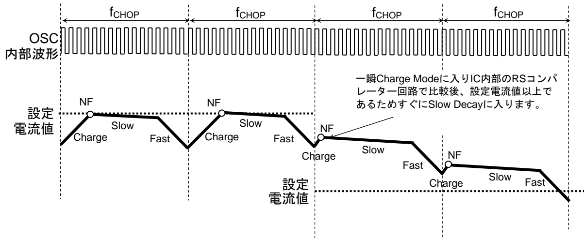
図 7.11.3 設定電流値が減少方向の場合
