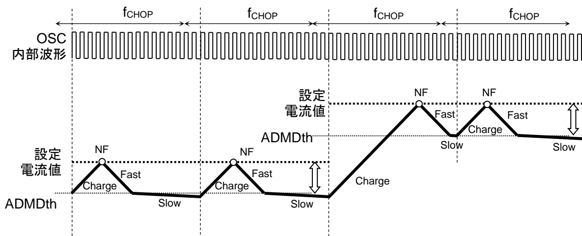
図 7.14.1 設定電流値が増加方向の場合
