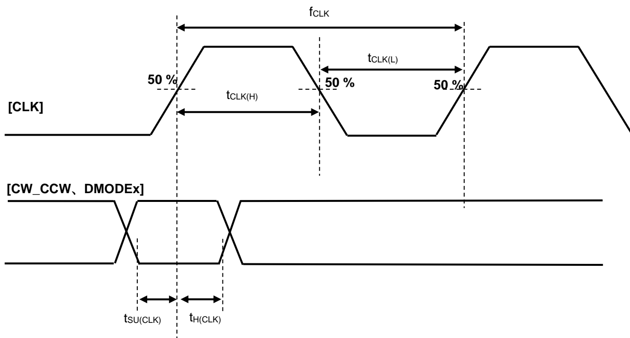
図 20.2 TB67S589FTG(CLK とその他制御信号の関係)
