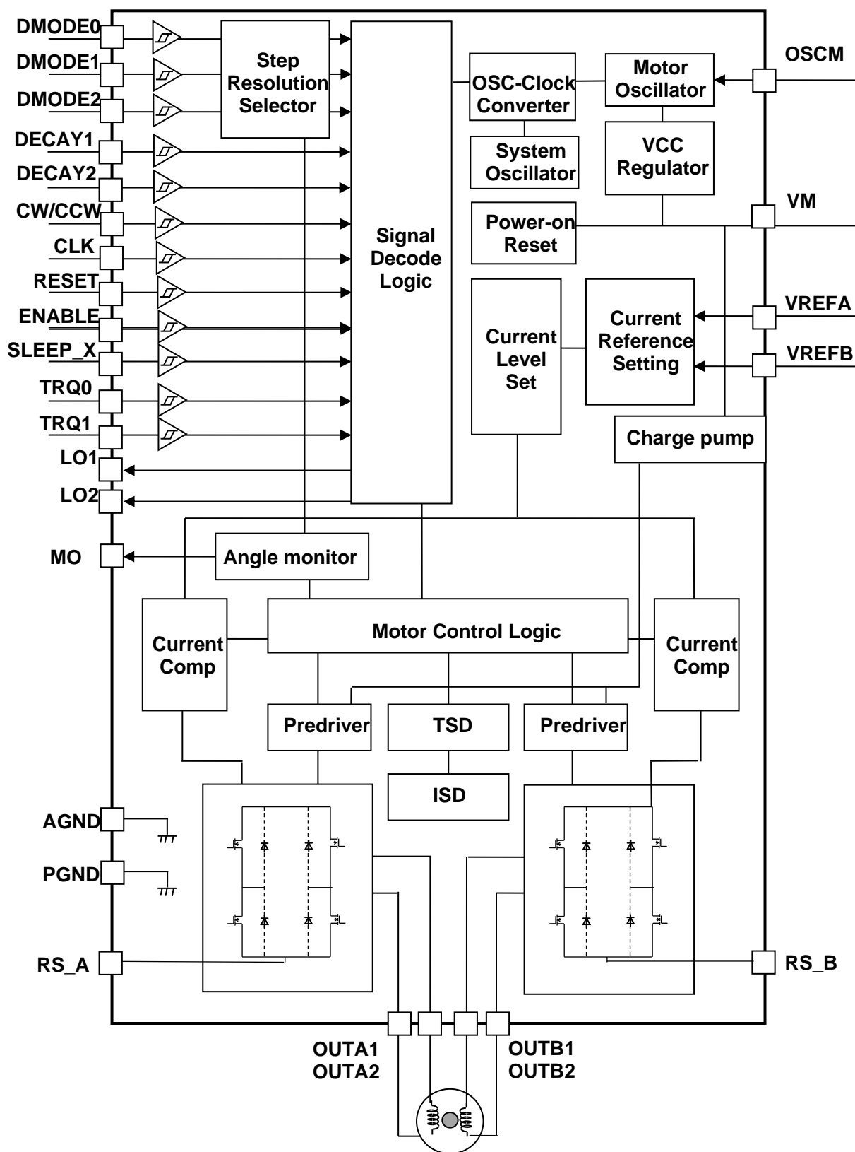
図4 ブロック図
