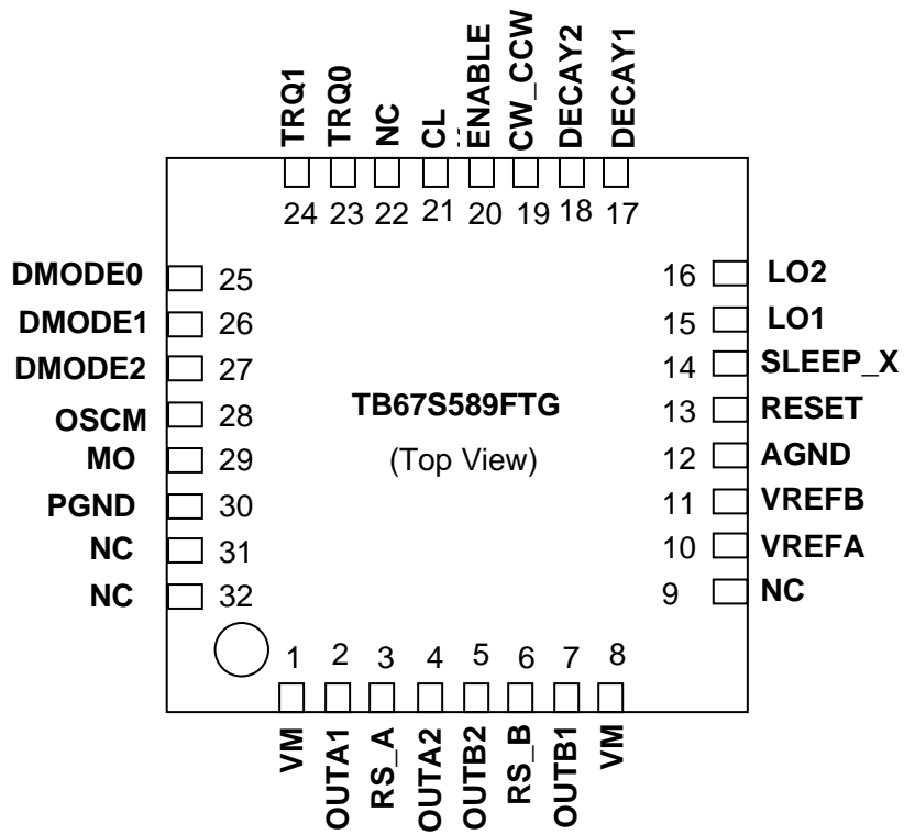
図3 ピン配置図
