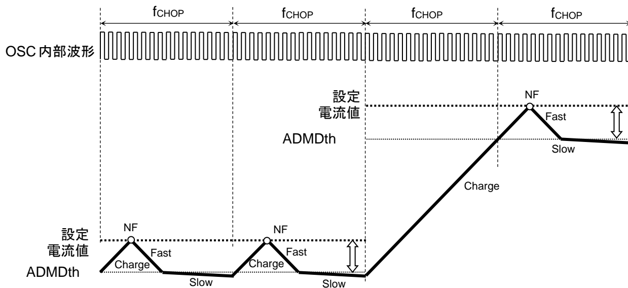
図 7.14.2 Charge 期間が f_{CHOP} 1 周期以上の場合
