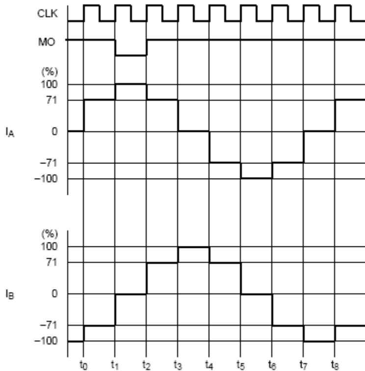
1/2-步励磁模式(A型) (M1: L, M2: H, M3: L, CW 模式)
