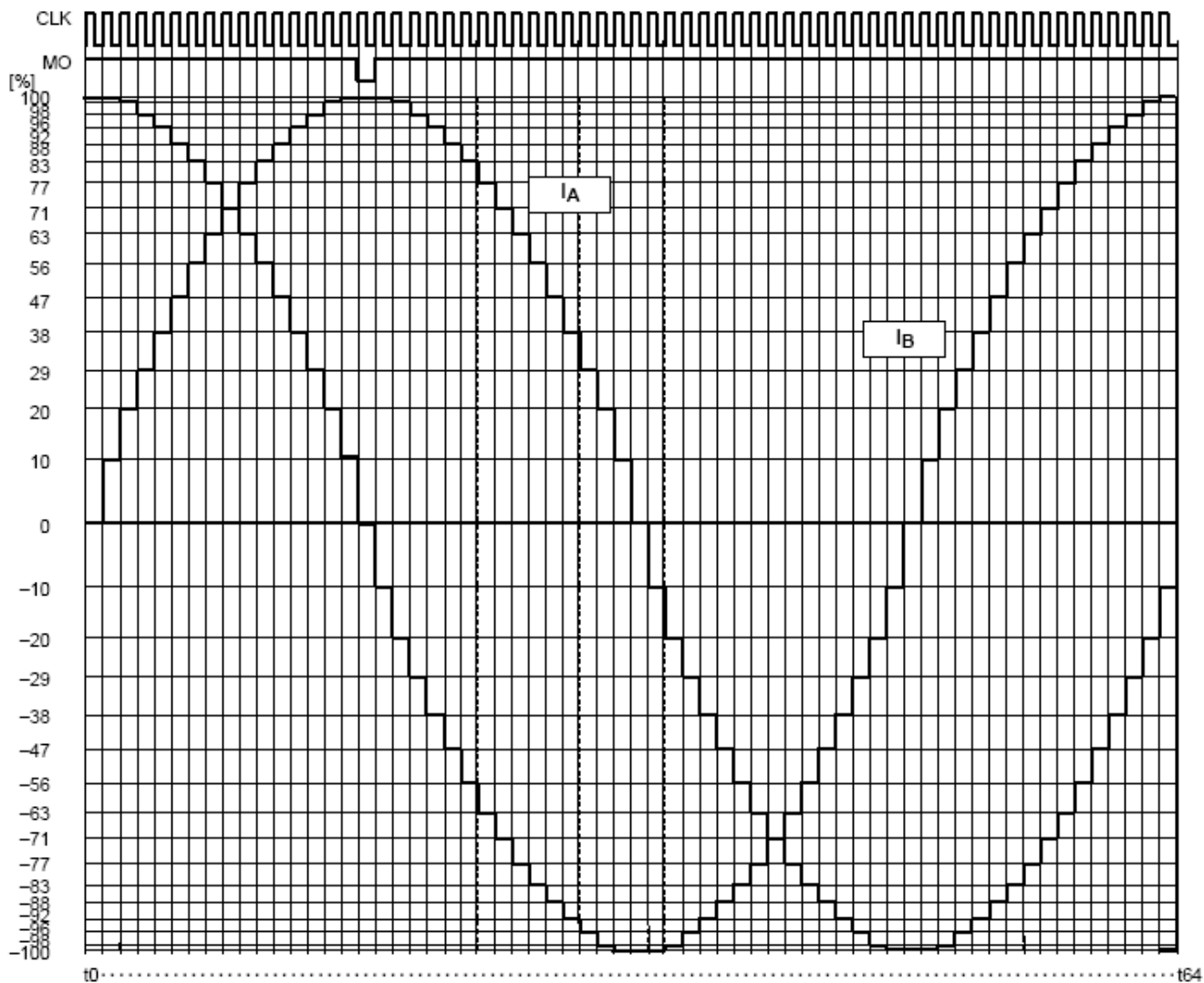
1/16-步励磁模式(M1: H, M2: H, M3: L, CCW 模式)
