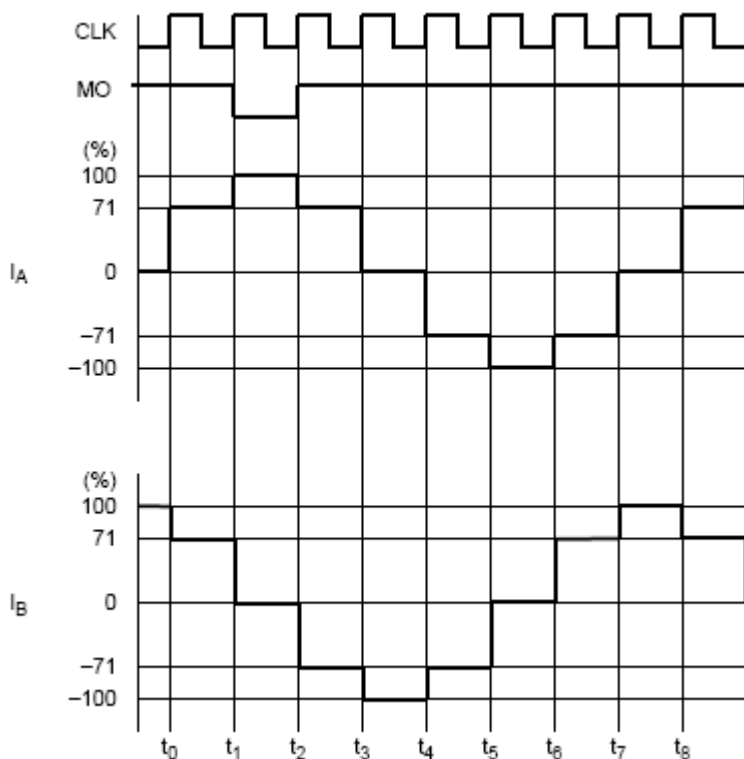
1/2-步励磁模式(A型) (M1: L, M2: H, M3: L, CCW 模式)
