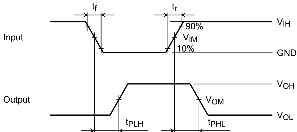
図 11.8.1 t_{PLH} , t_{PHL}
