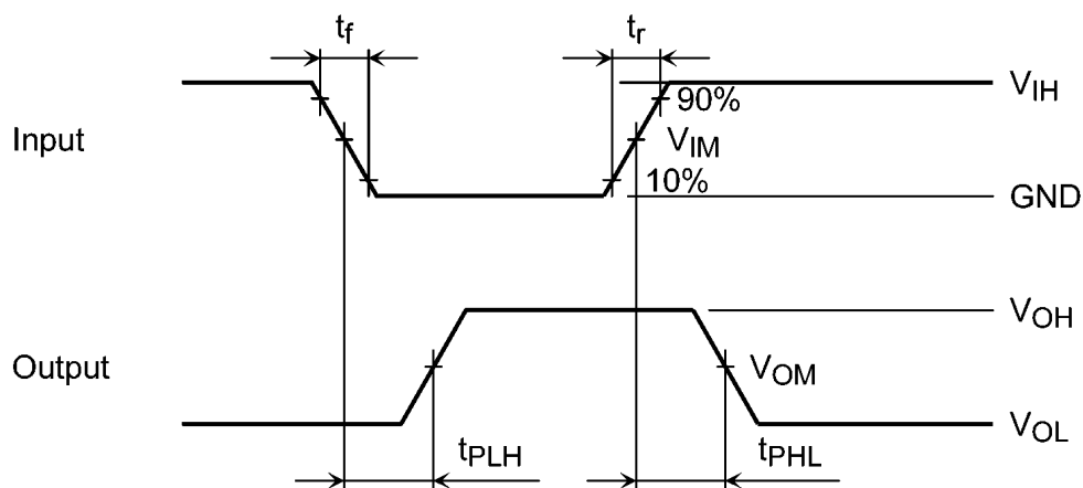
図 11.8.1 t_{PLH} , t_{PHL}
