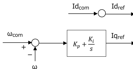
図 6 速度制御ブロック図
