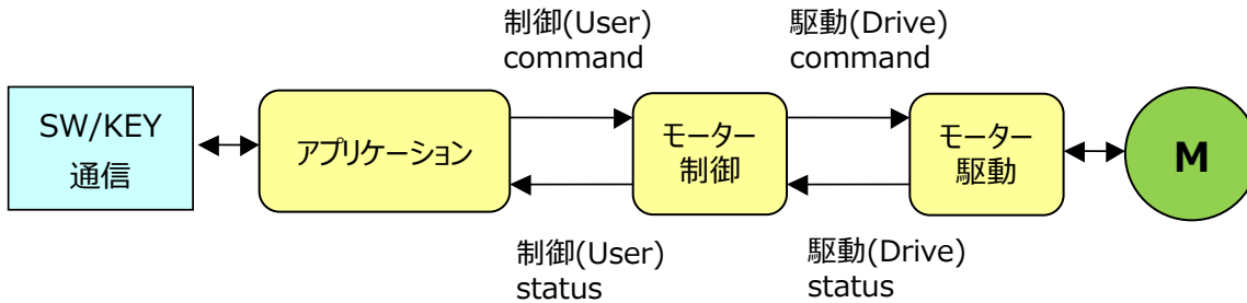
図 1 ベクトル制御ソフトウェアの構造
