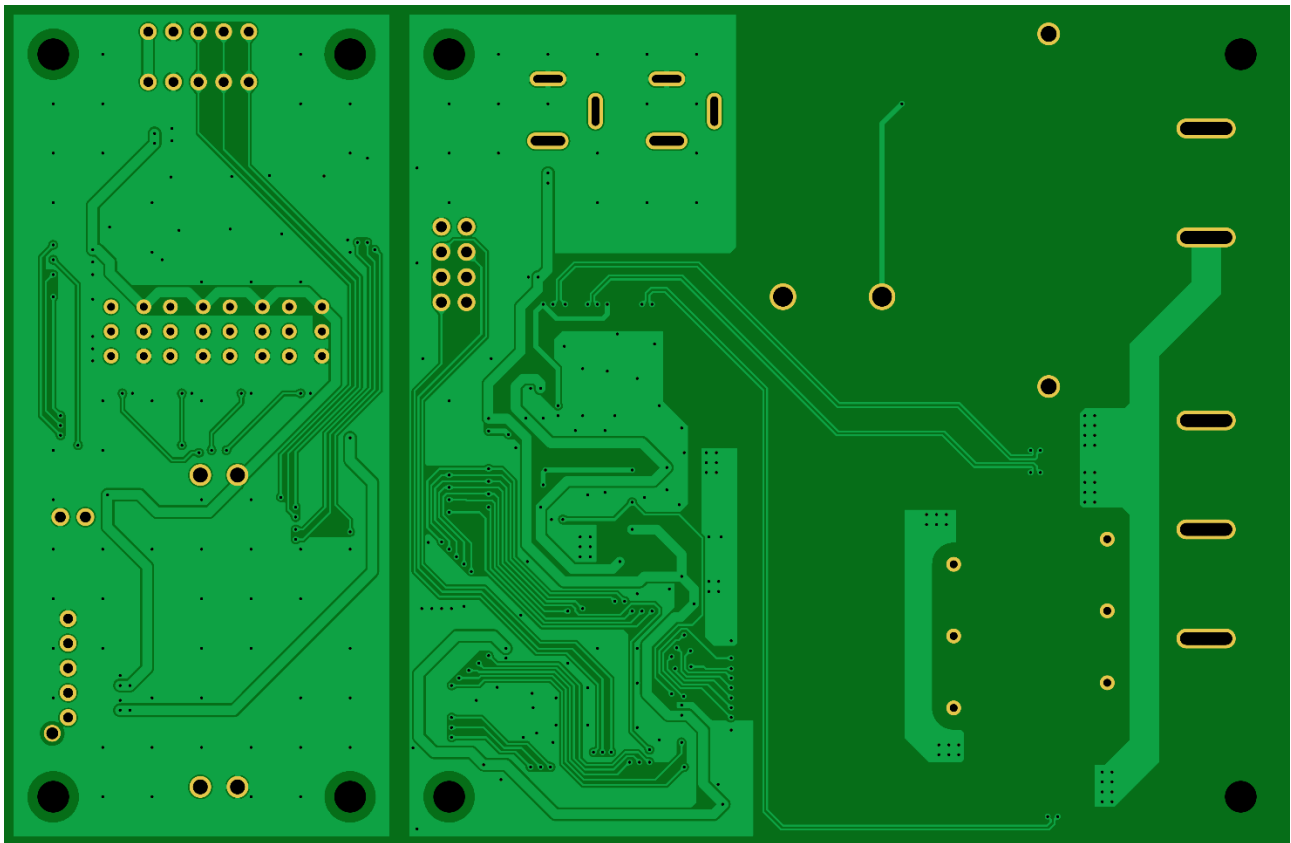
図 2.4 主要部品配置 (RD179-1, Back 側)
