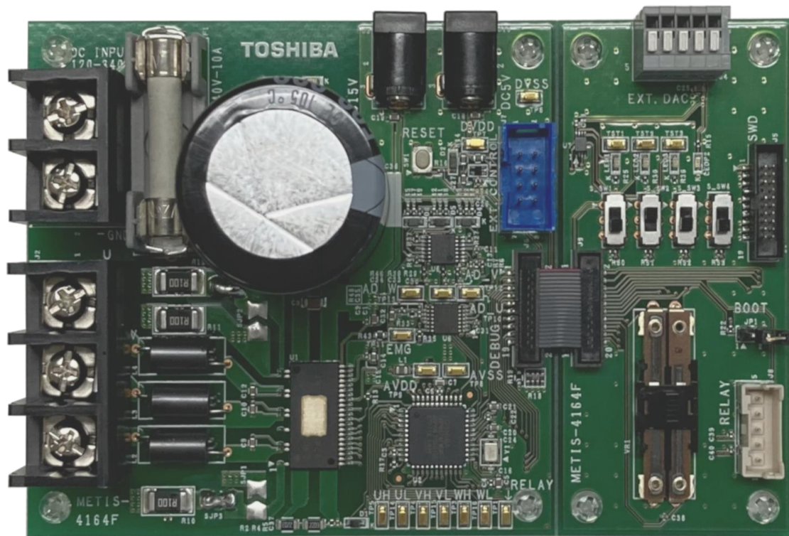
図 2.2 DC300 V 入カブラシレス DC モーターセンサーレス駆動回路 基板正面図(RD179-1)
