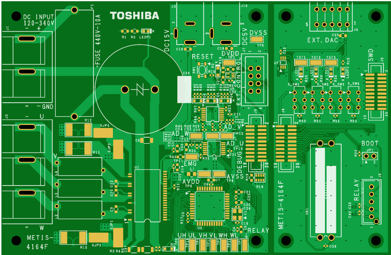
図 2.3 主要部品配置 (RD179-1, Front 側)
