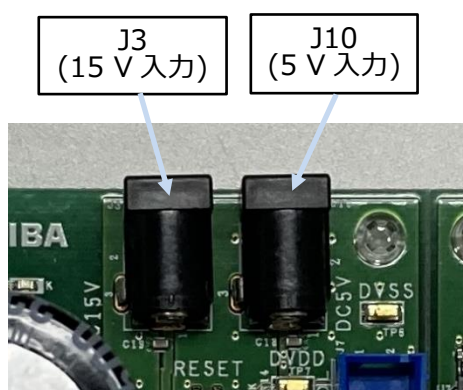
図 4.4 基板上的制御電源入力端子(J3, J10)
