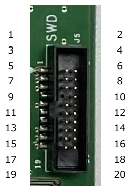
図 4.10 デバッガーコネクタ(J5)
