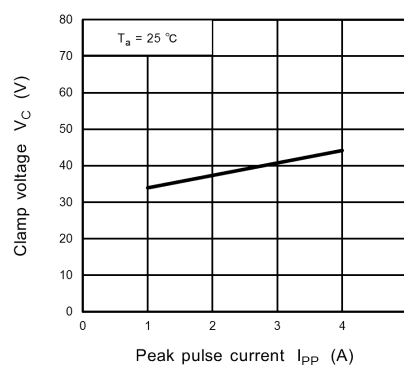
Fig. 10.19.2 V_C - I_{PP}
