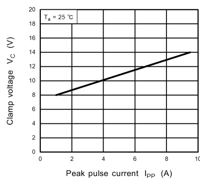
Fig. 10.5.2 V_C - I_{PP}
