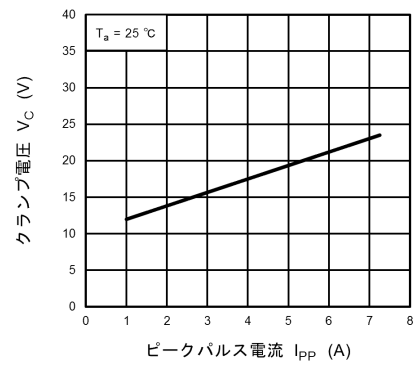
図 10.9.2 V_C - I_{PP}
