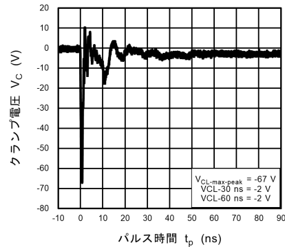
図 10.7.6 ISO10605 クランプ波形 -8 kV
