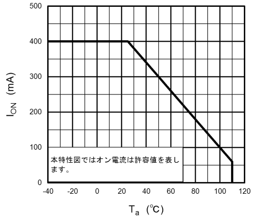
図 12.2 I_{ON} - T_a
