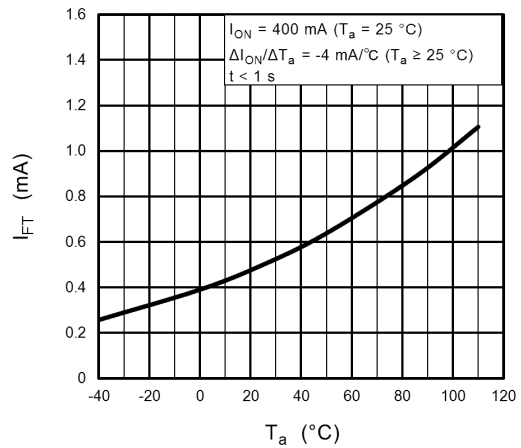
図 12.6 I_{FT} - T_a
