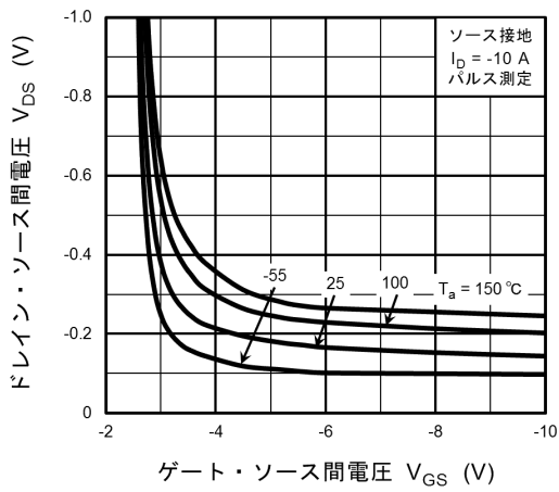
図 8.3 V_{DS} - V_{GS}
