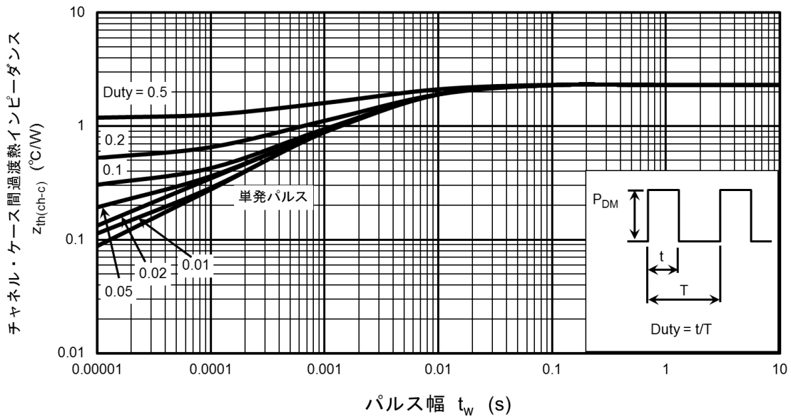
図 8.15 Z_{th(ch-c)} - t_w (最大値 (保証値))
