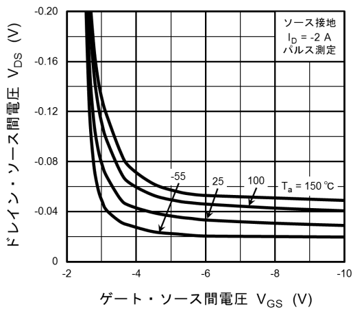
図 8.5 V_{DS} - V_{GS}
