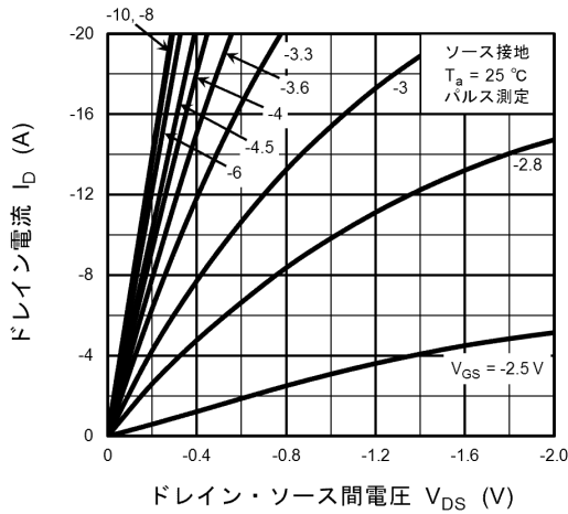
図 8.1 I_D - V_{DS}
