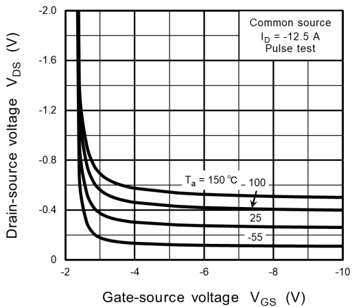
Fig. 8.3 V_{DS} - V_{GS}
