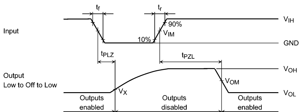
図 12.8.1 t_{PLH} , t_{PHL}
