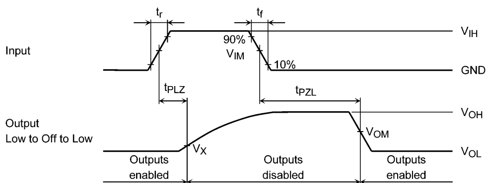
図 12.8.1 t_{PLZ} , t_{PZL}
