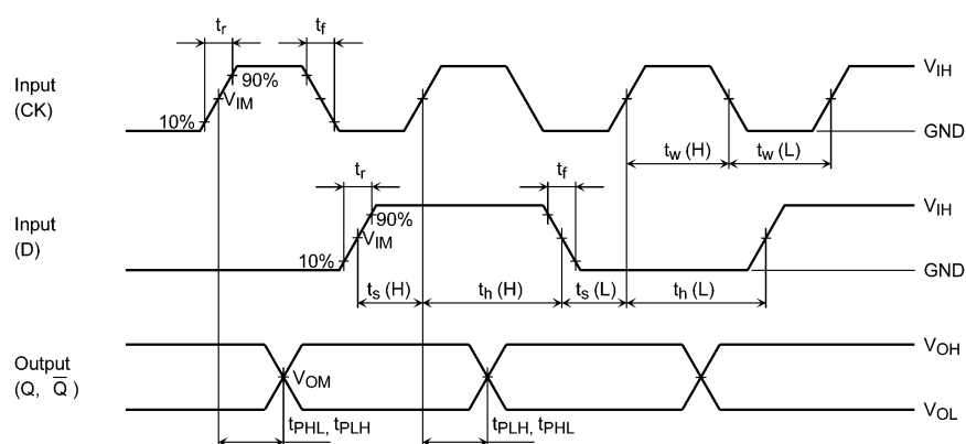
図 11.8.1 t_{PLH} , t_{PHL} , t_w , t_s , t_h
