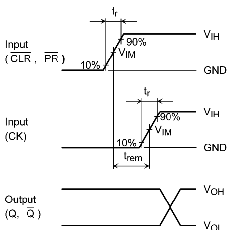
図 11.8.2 t_{rem}
