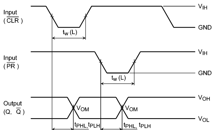
図 11.8.3 t_{PLH} , t_{PHL}
