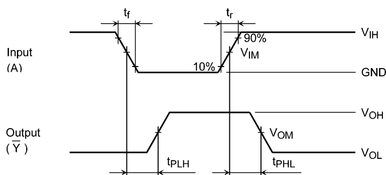
図 11.6.1 t_{PLH} , t_{PHL}
