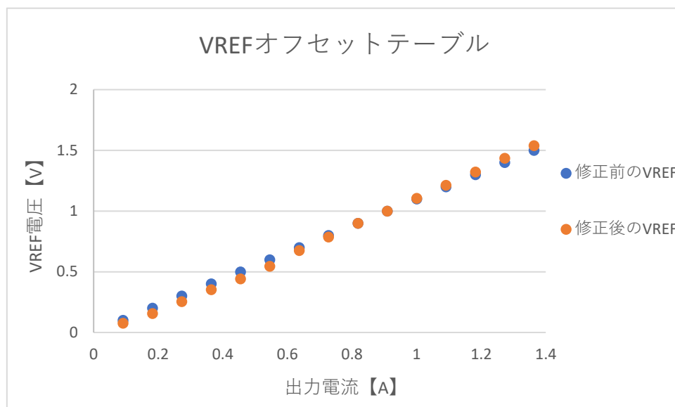
図 4.1 VREF オフセットテーブル
