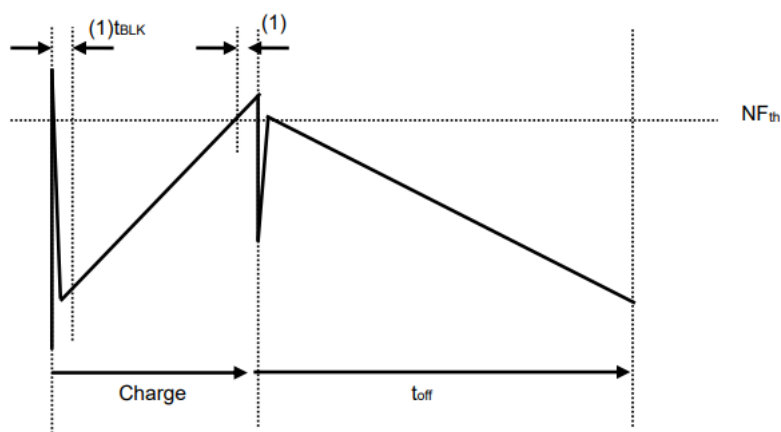
図 4.2 定電流 PWM タイミングチャート
