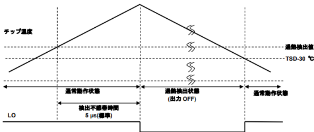
図 5.1 過熱検出のタイミングチャート 1
