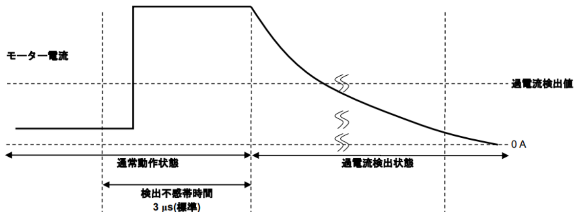
図 5.3 過電流検出タイミングチャート
