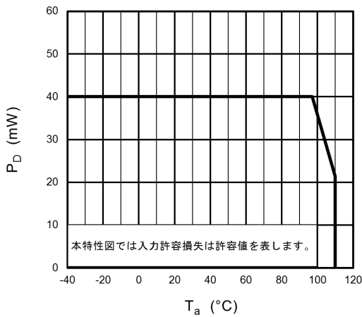
図 14.3 P_D - T_a
