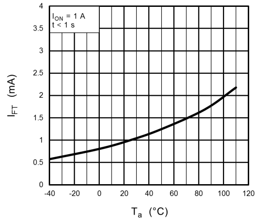
图 14.8 I_{FT} - T_a
