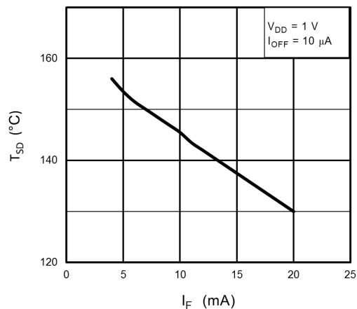
図 14.14 T_{SD} - I_F
