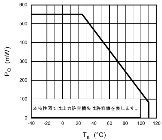
図 14.4 P_O - T_a
