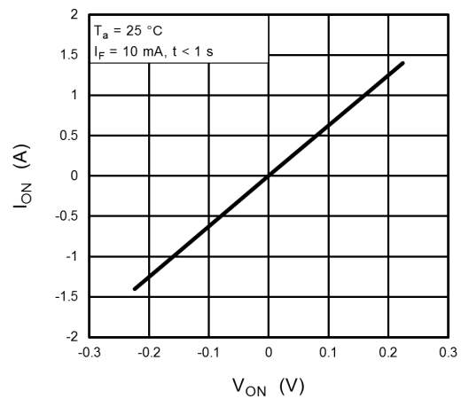
図 14.6 I_{ON} - V_{ON}
