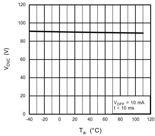
図 14.15 V_{OVC} - T_a
