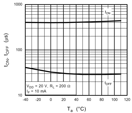
图 14.10 t_{ON}, t_{OFF} - T_a
