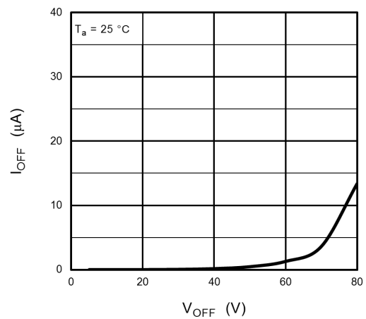
图 14.12 I_{OFF} - V_{OFF}
