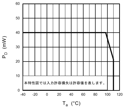
図 14.3 P_D - T_a
