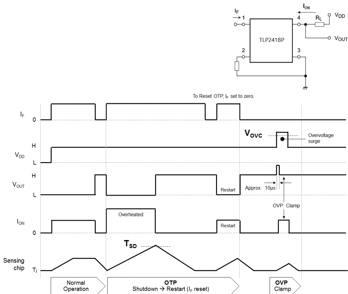
図 15.3.1 タイミングチャート
