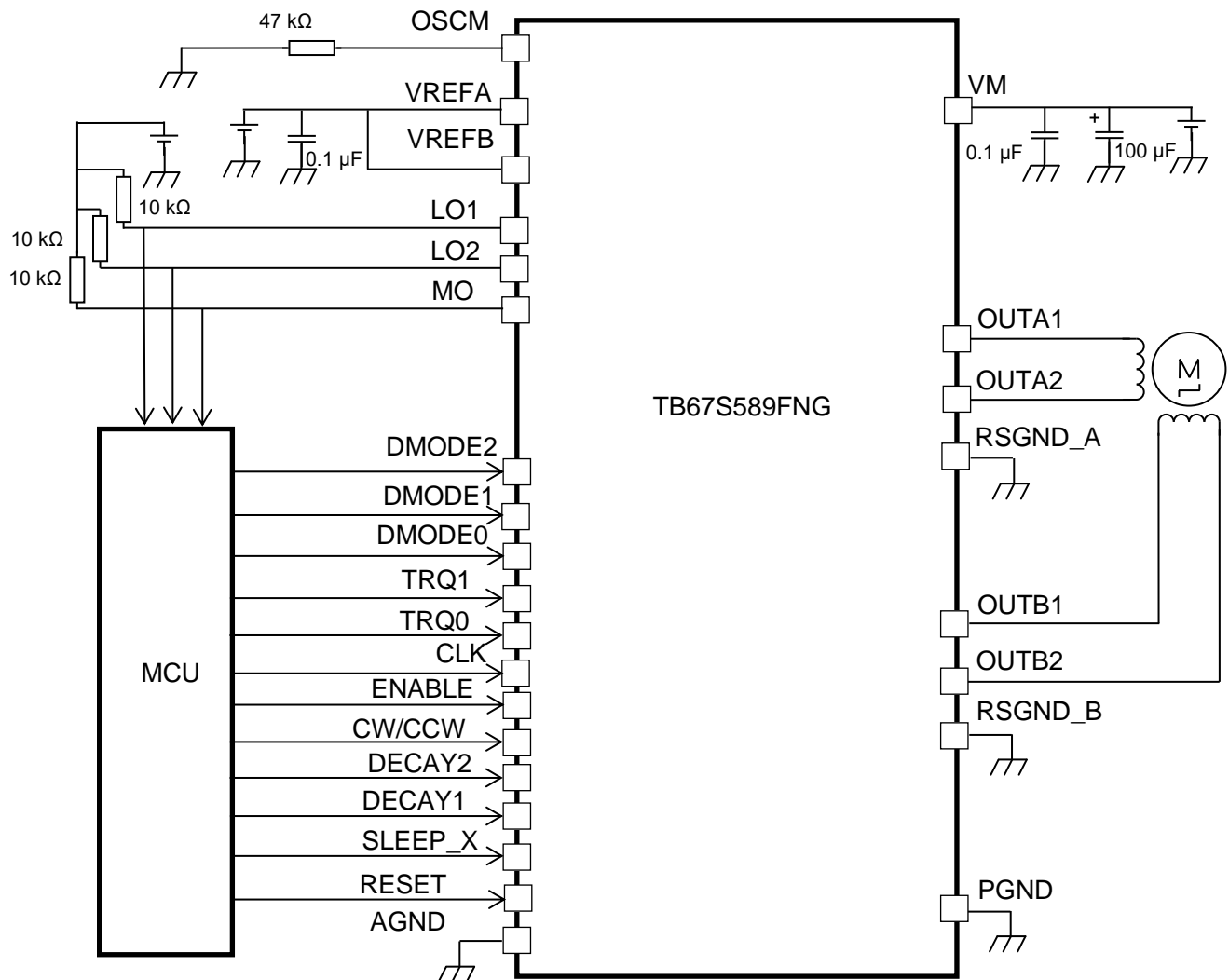
図 7.1 応用回路例
