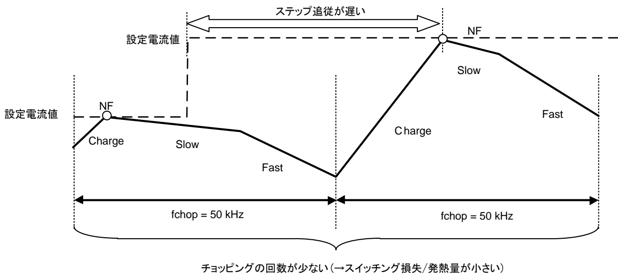
図 4.2 定電流波形 ( f_{chop} = 50 \text{ kHz} の場合)
