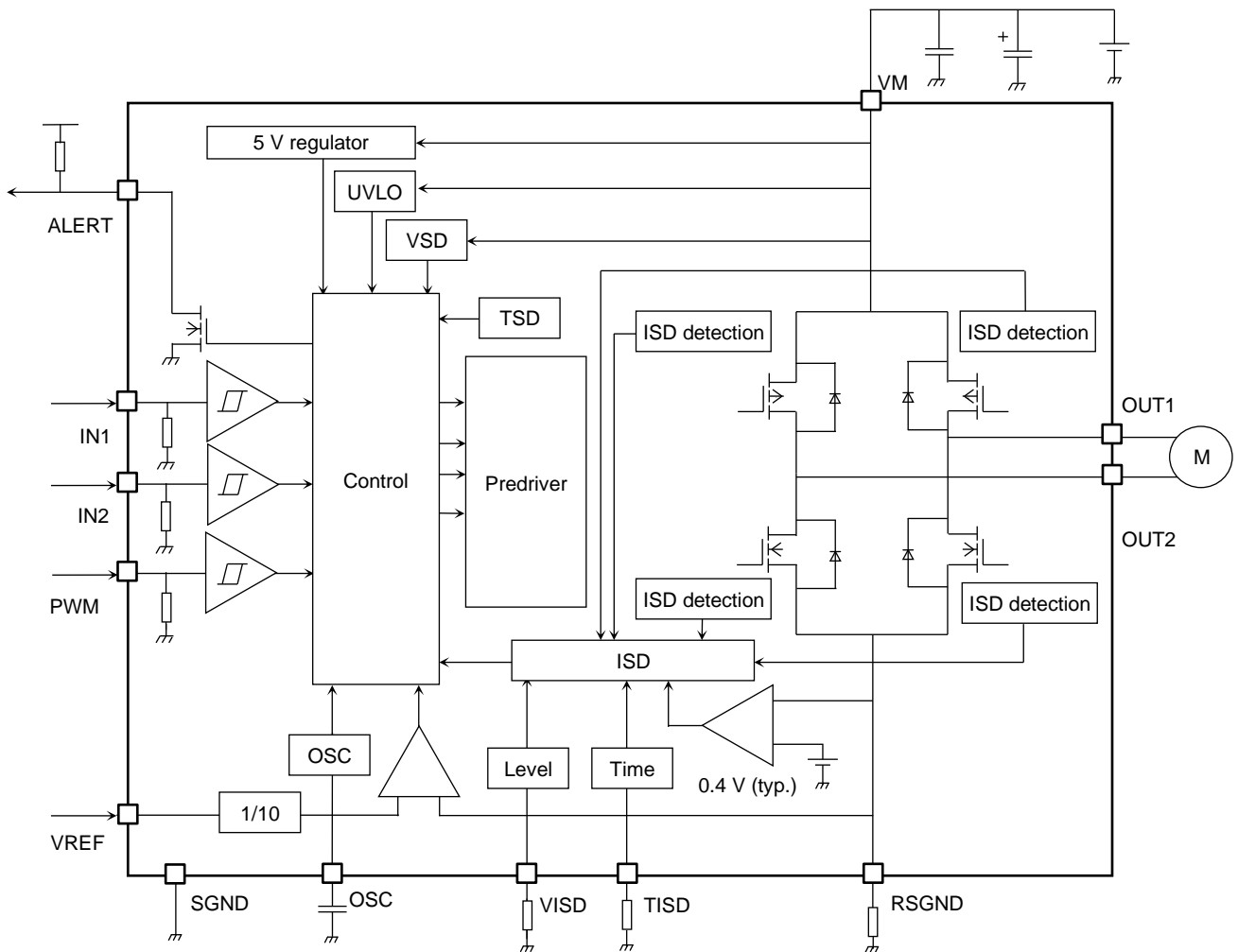
図3 ブロック図
