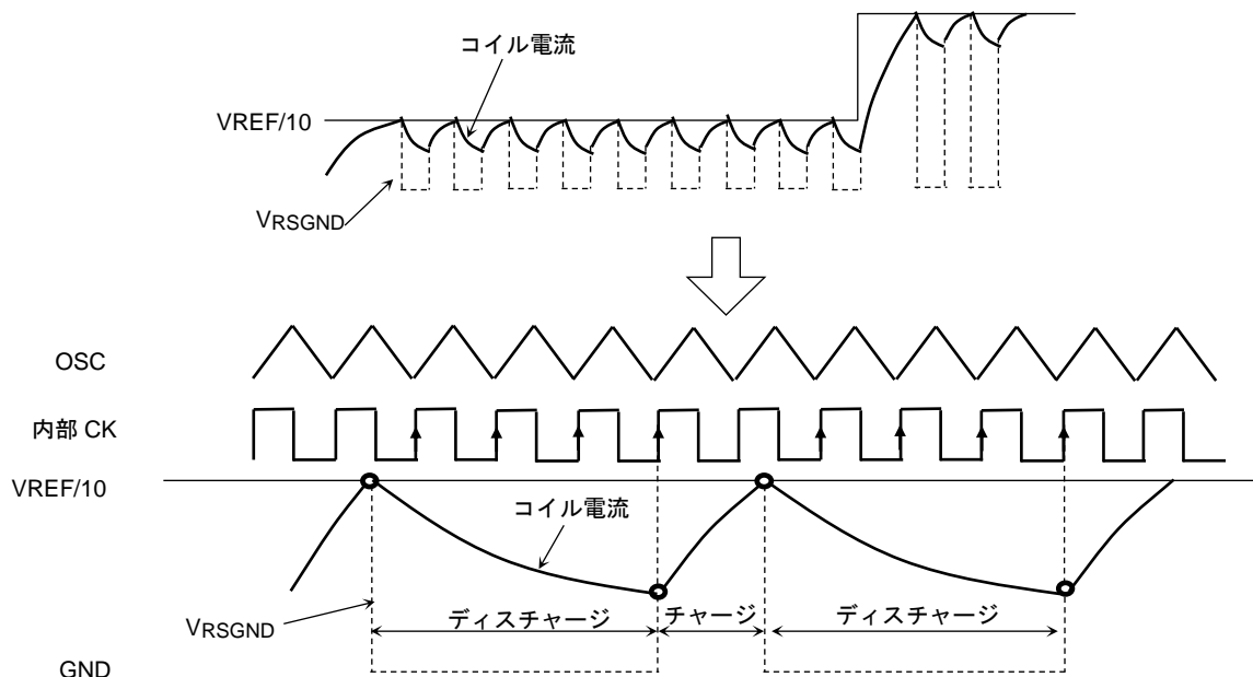
図 13.9.2 定電流チョッピング
