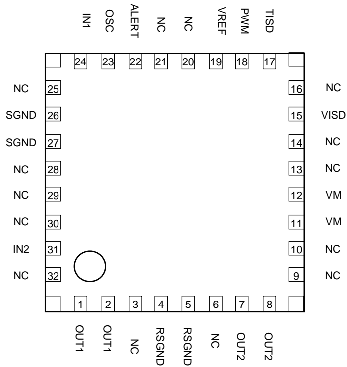
图 7 TB6569FTG 端子配置图
