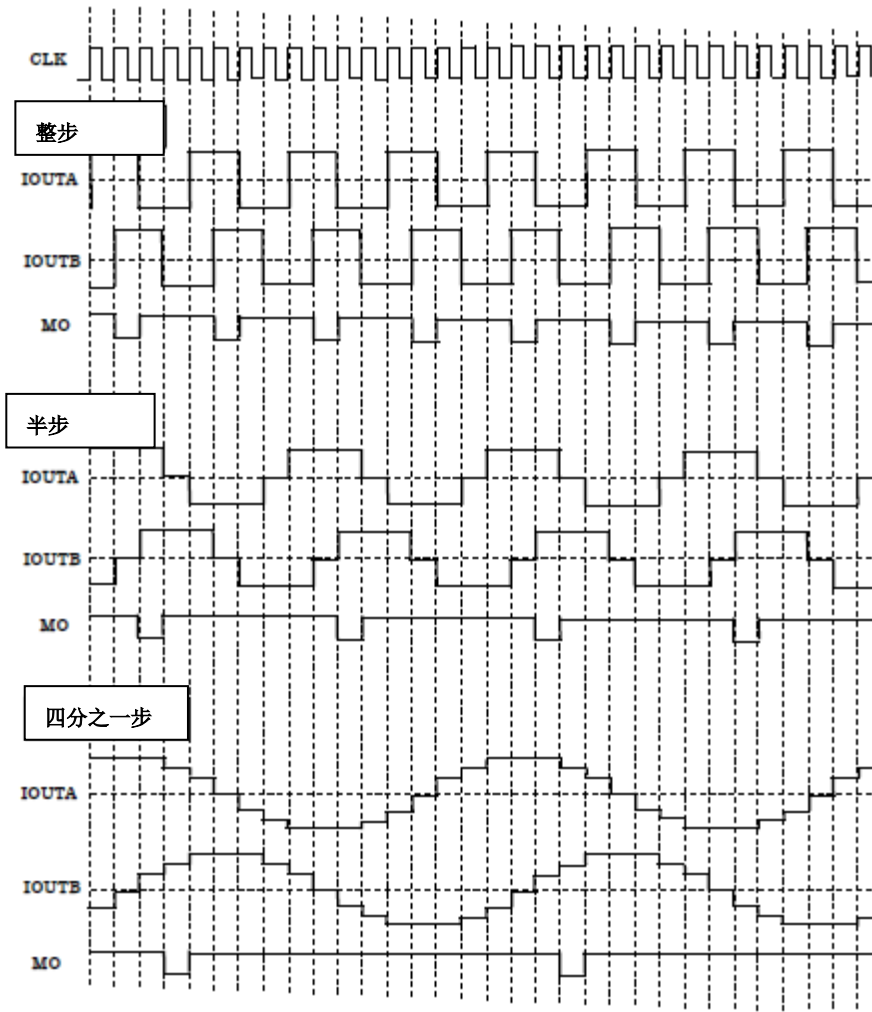
步数分辨率时序图 (CLK-IN)
