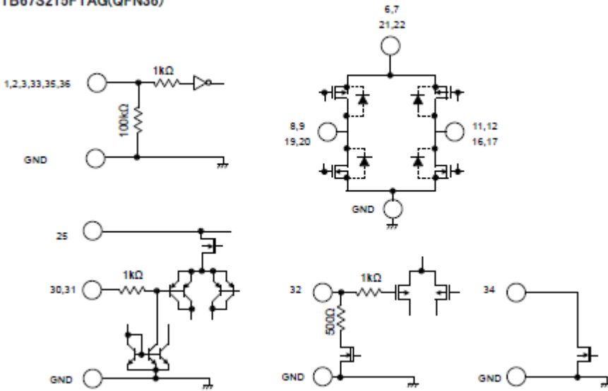
TB67S215FTAG(QFN36)
