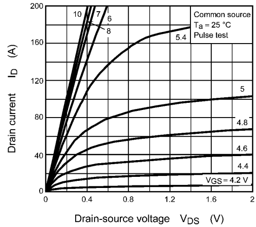
Fig. 9.2 I_D - V_{DS}
