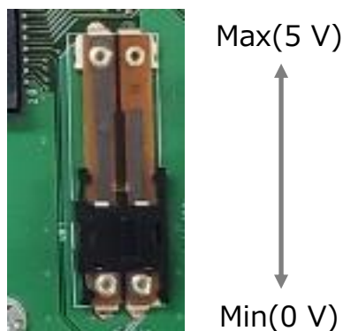
図 4.6 基板上のポテンシオメータ(VR1)
