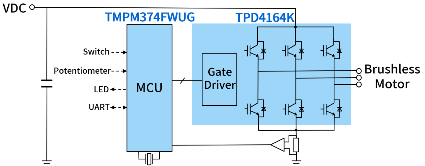
図 2.1 DC300 V 入力ブラシレス DC モーターセンサーレス駆動回路ブロック図
