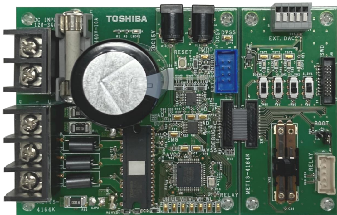
図 2.2 DC300 V 入カブラシレス DC モーターセンサーレス駆動回路 基板正面図(RD179-2)
