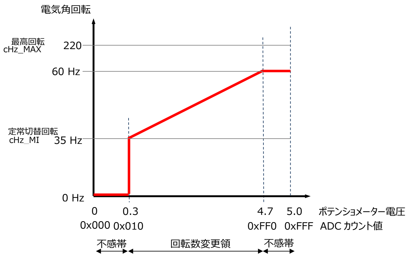
図 4.7 ポテンシオメータ設定値と回転速度との関係
