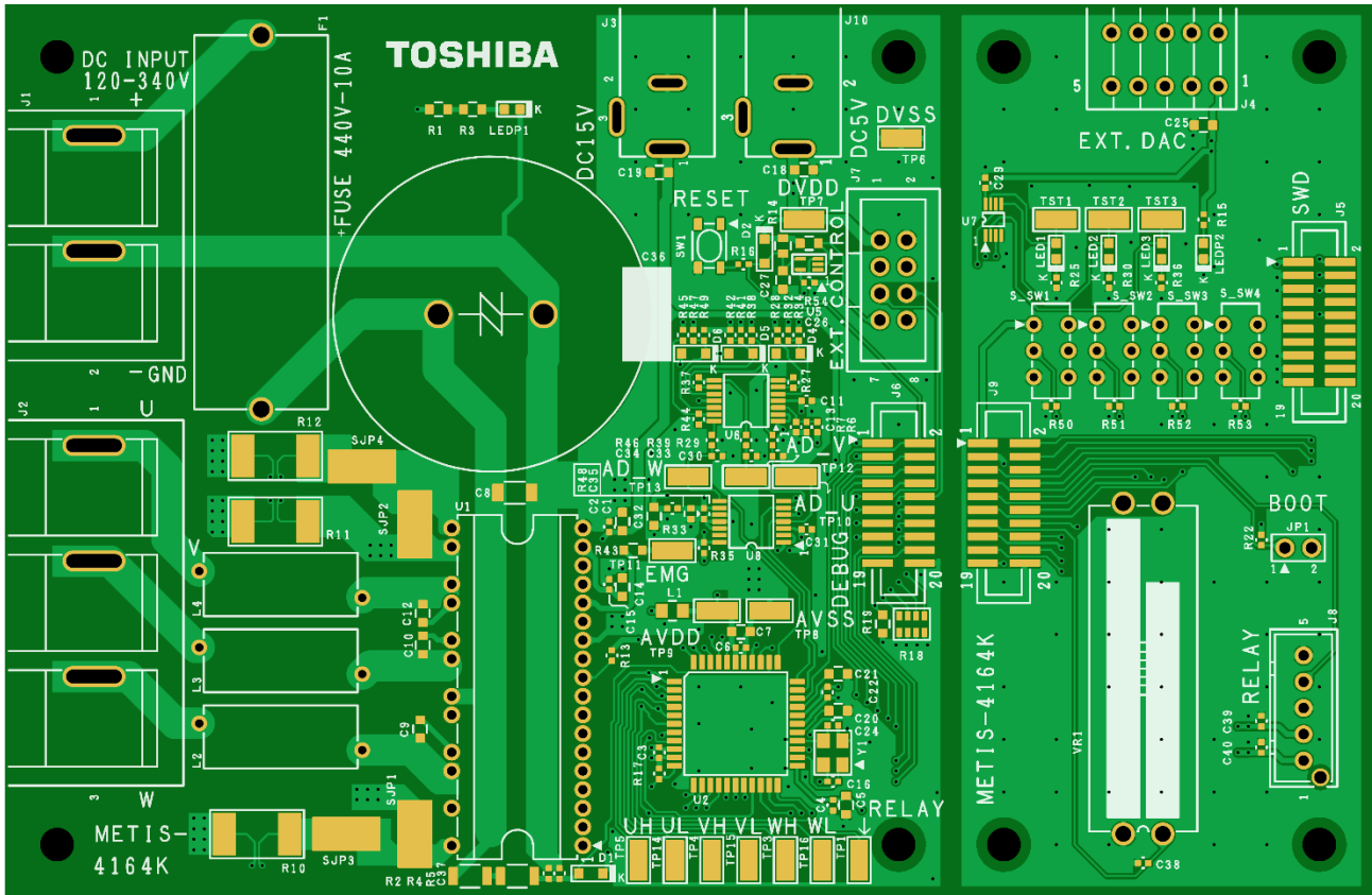
図 2.3 主要部品配置 (RD179-2, Front 側)
