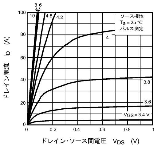
図 9.1 I_D - V_{DS}
