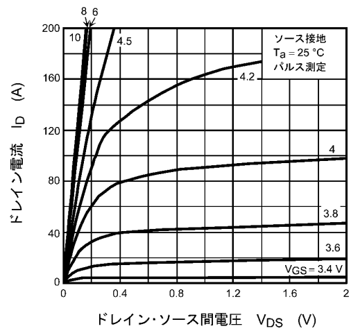
図 9.2 I_D - V_{DS}
