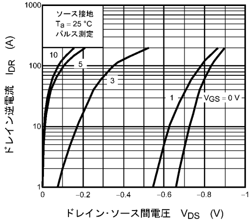
図 9.7 I_{DR} - V_{DS}
