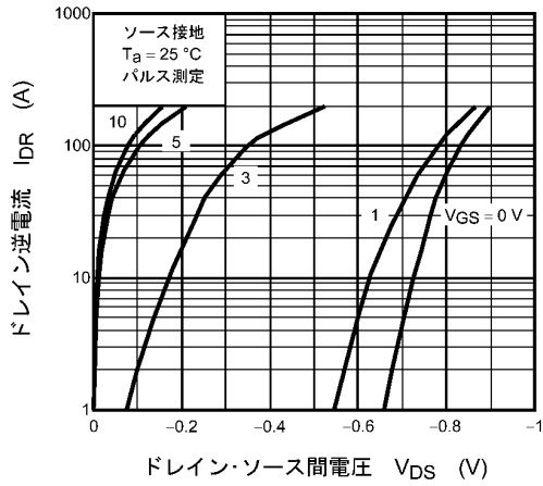
図 9.7 I_{DR} - V_{DS}
