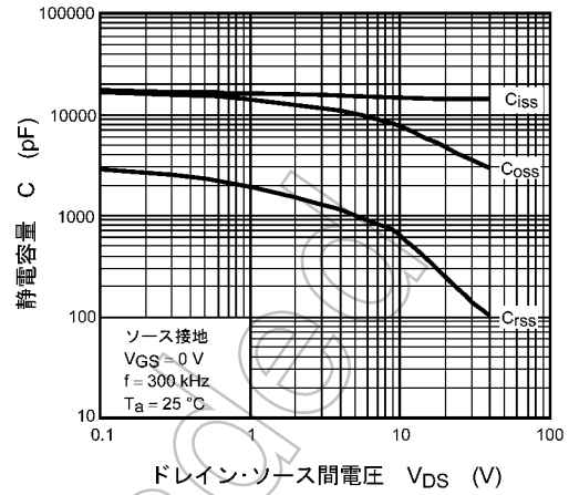
図 9.8 静電容量 - V_{DS}
