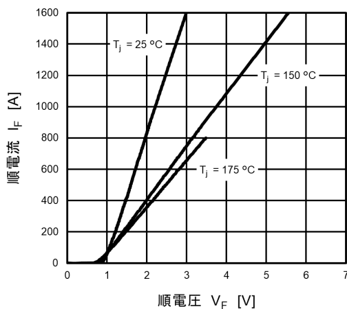
図 9.1 I_F - V_F (注1)
