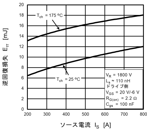
図 8.9 E_{rr} - I_S
