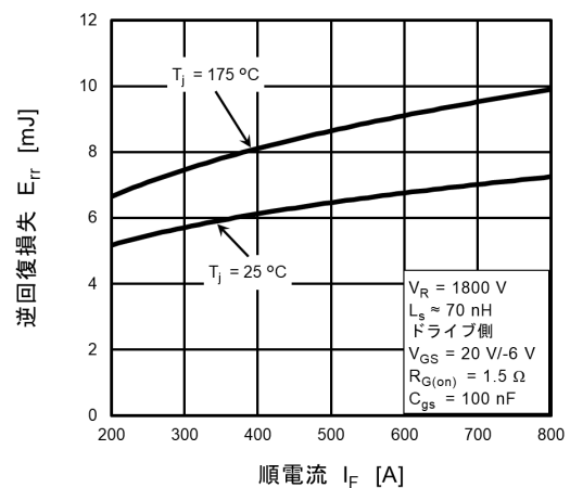
図 9.2 E_{rr} - I_F
